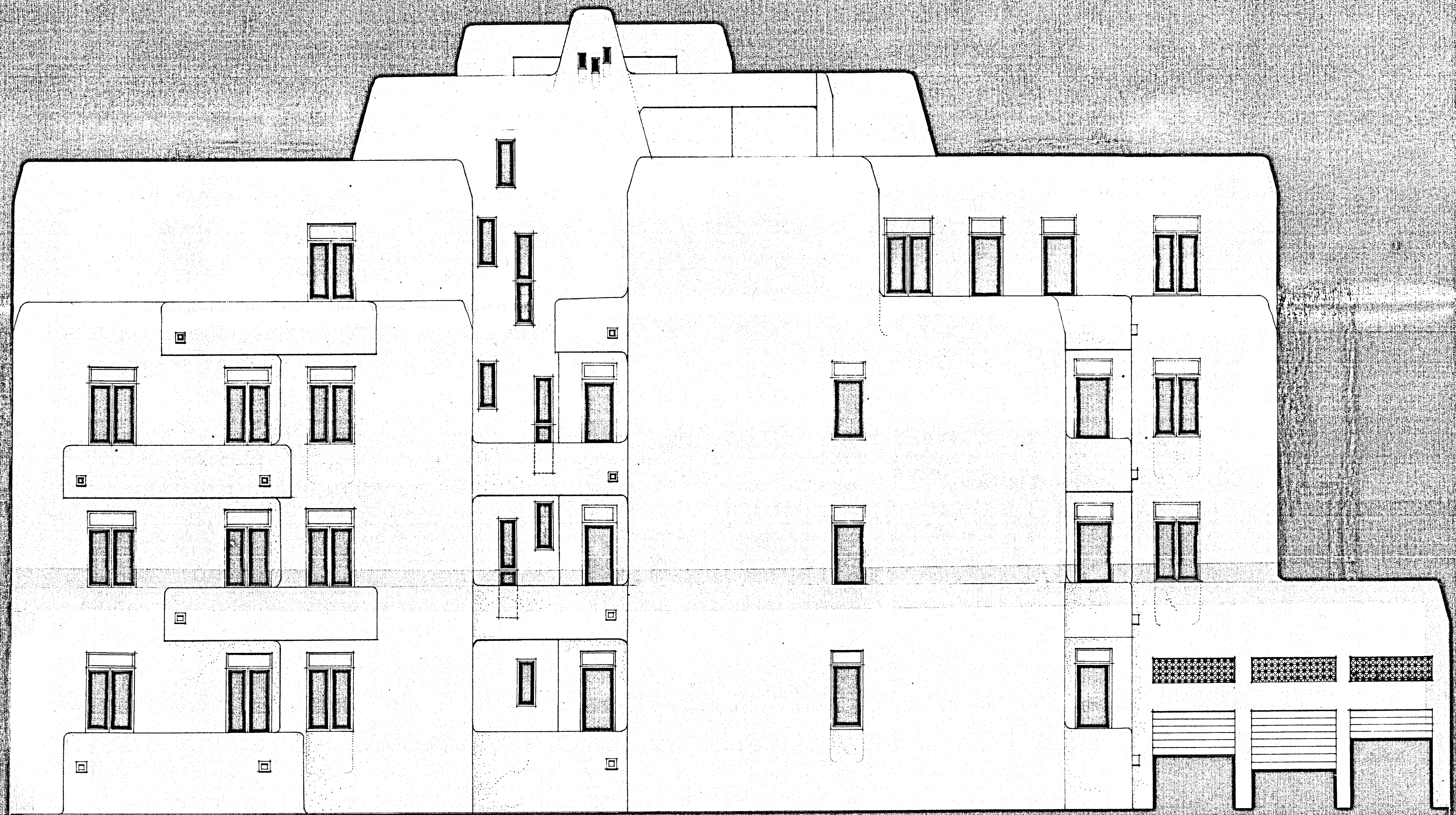
PROSPETTO -D-
