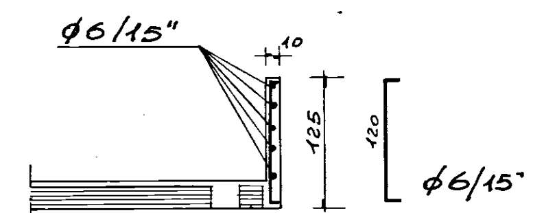
SEZ. A-A
