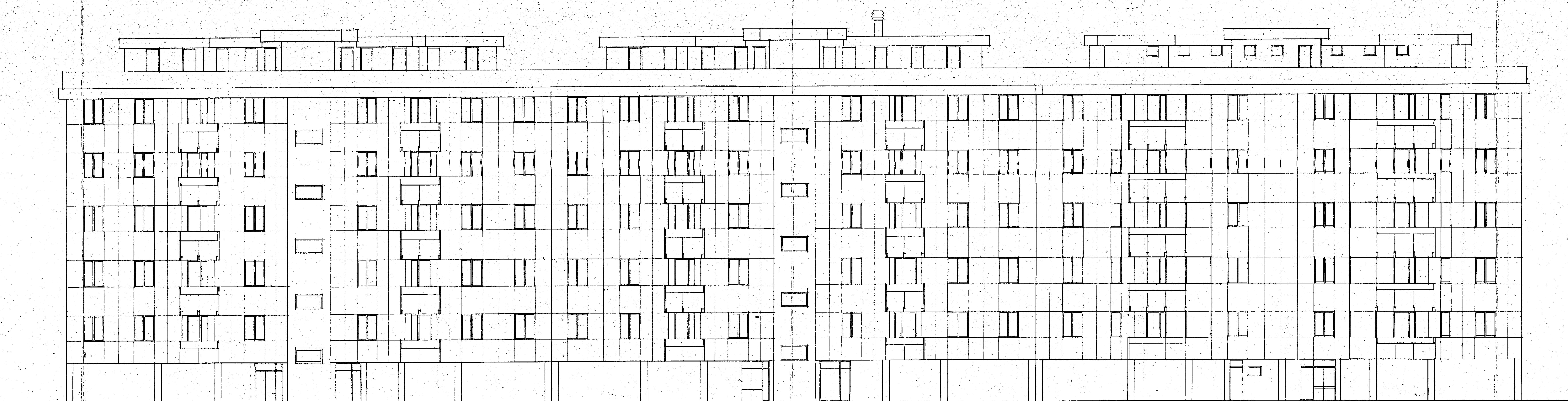
PROSPETTO b.
