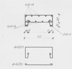
SEZIONE TRAVE DI CORONAMENTO PORTICO RALDI 1:20
