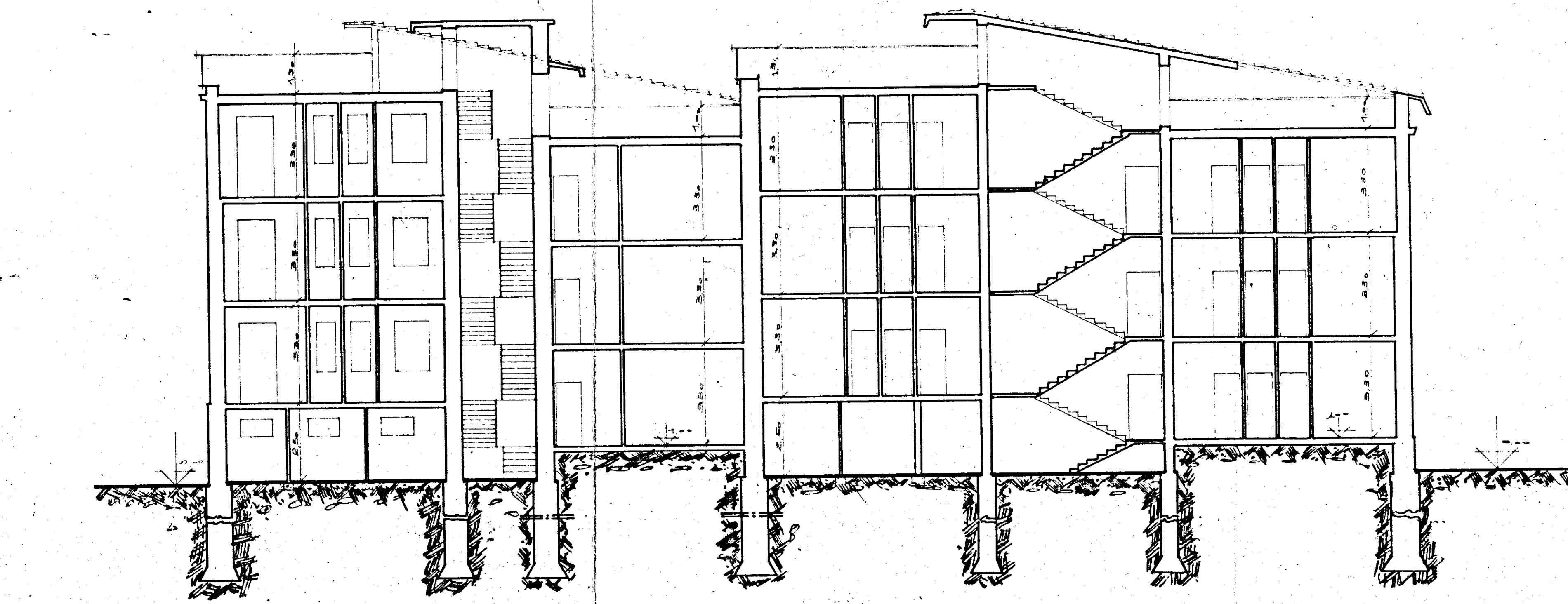
SEZIONE LONGITUDINALE
