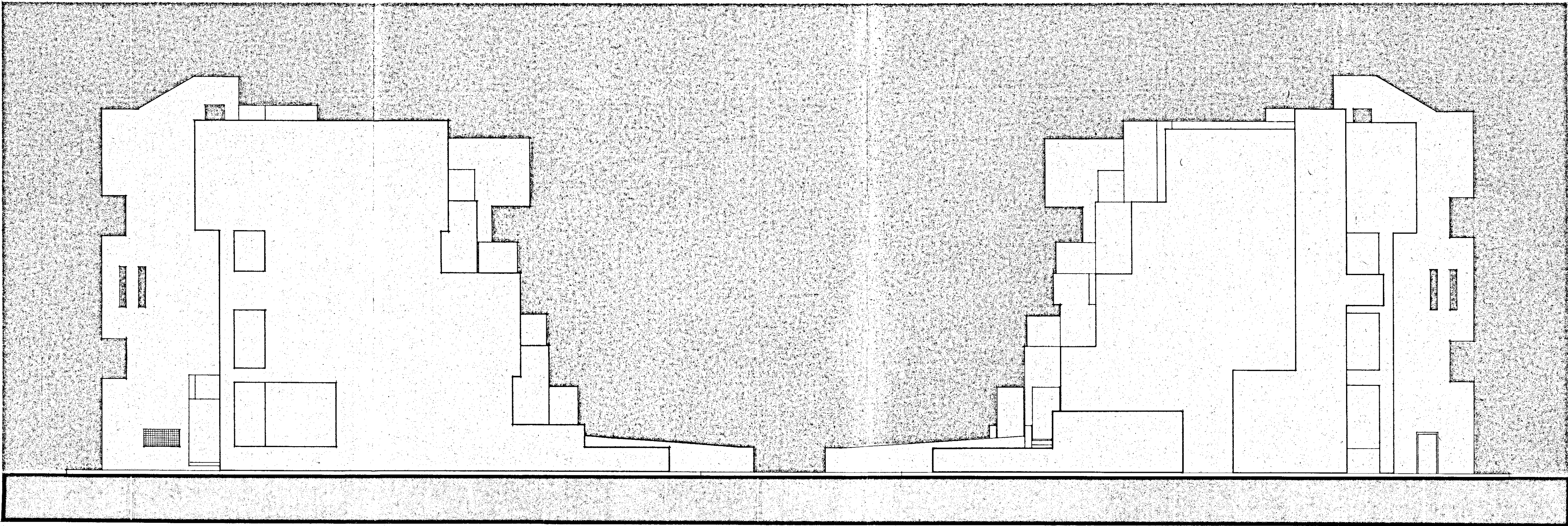
PROSPETTO 5-5
