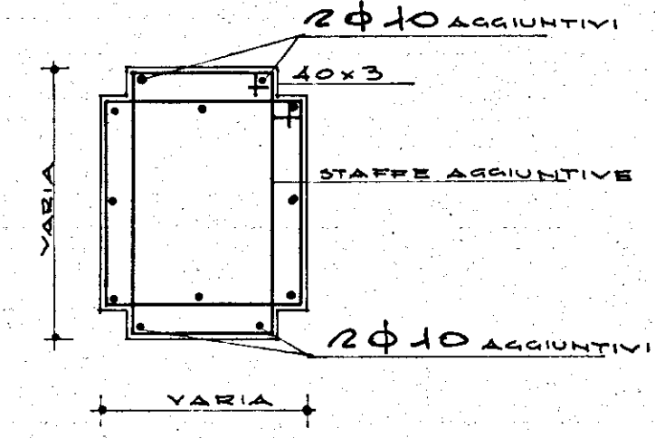
PARTICOLARE PILASTRI PORTICO 1:10
