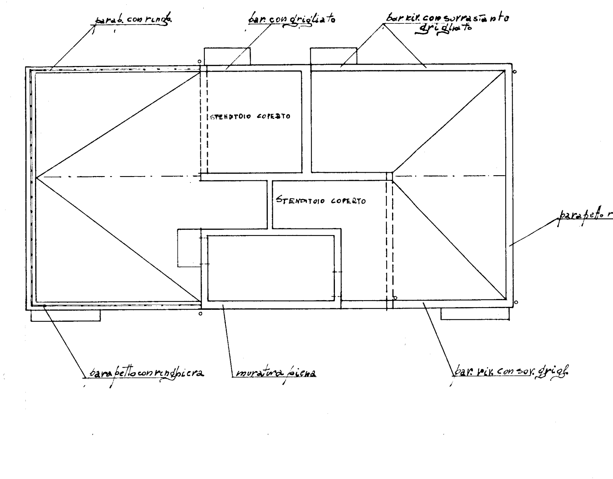
PIANTA TERRAZZA
