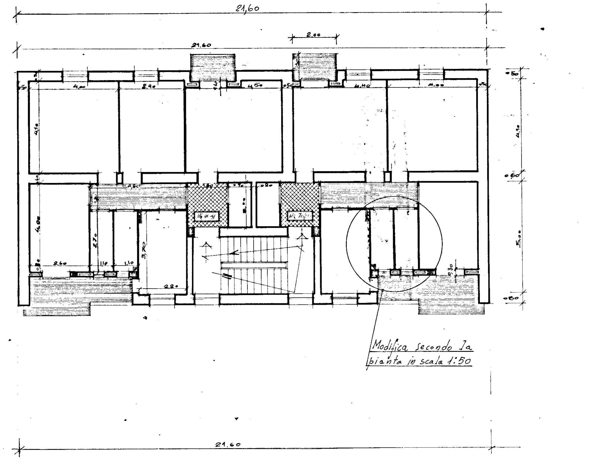
PRIMO PIANO
