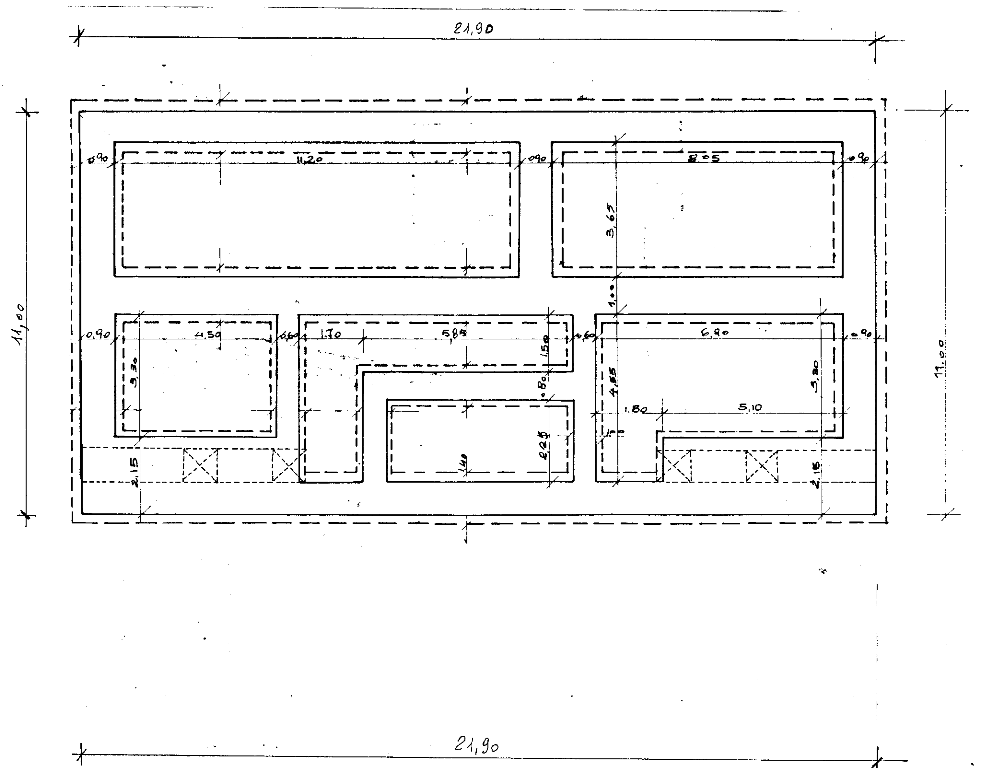
PIANTA FONDAZIONI
