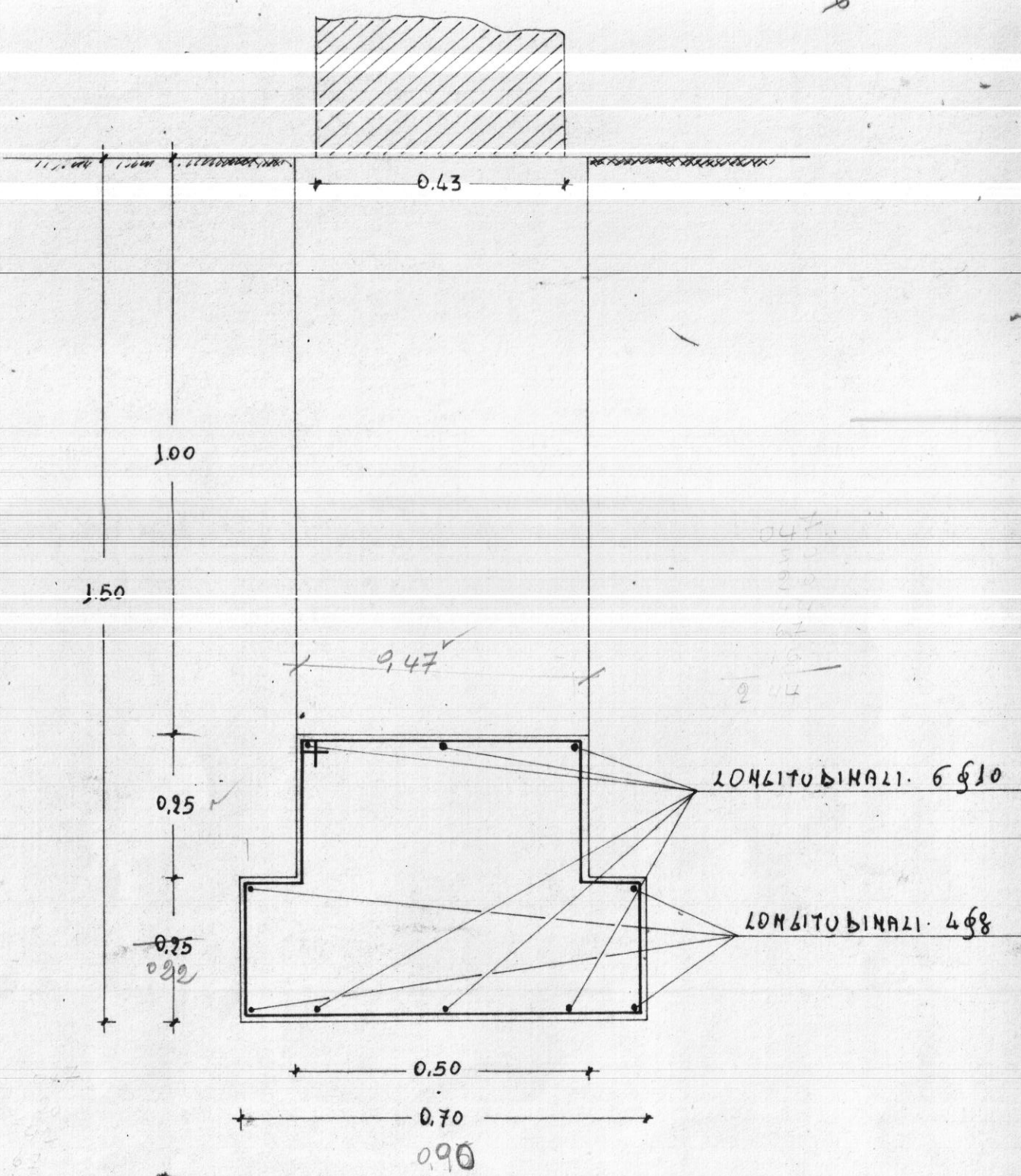
SEZIONI A-A'
