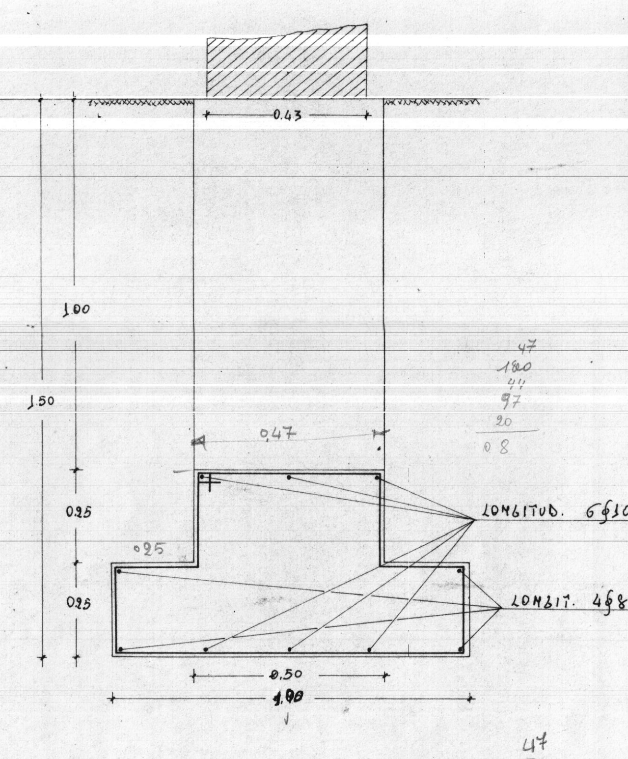
SEZIONI. C.C.
