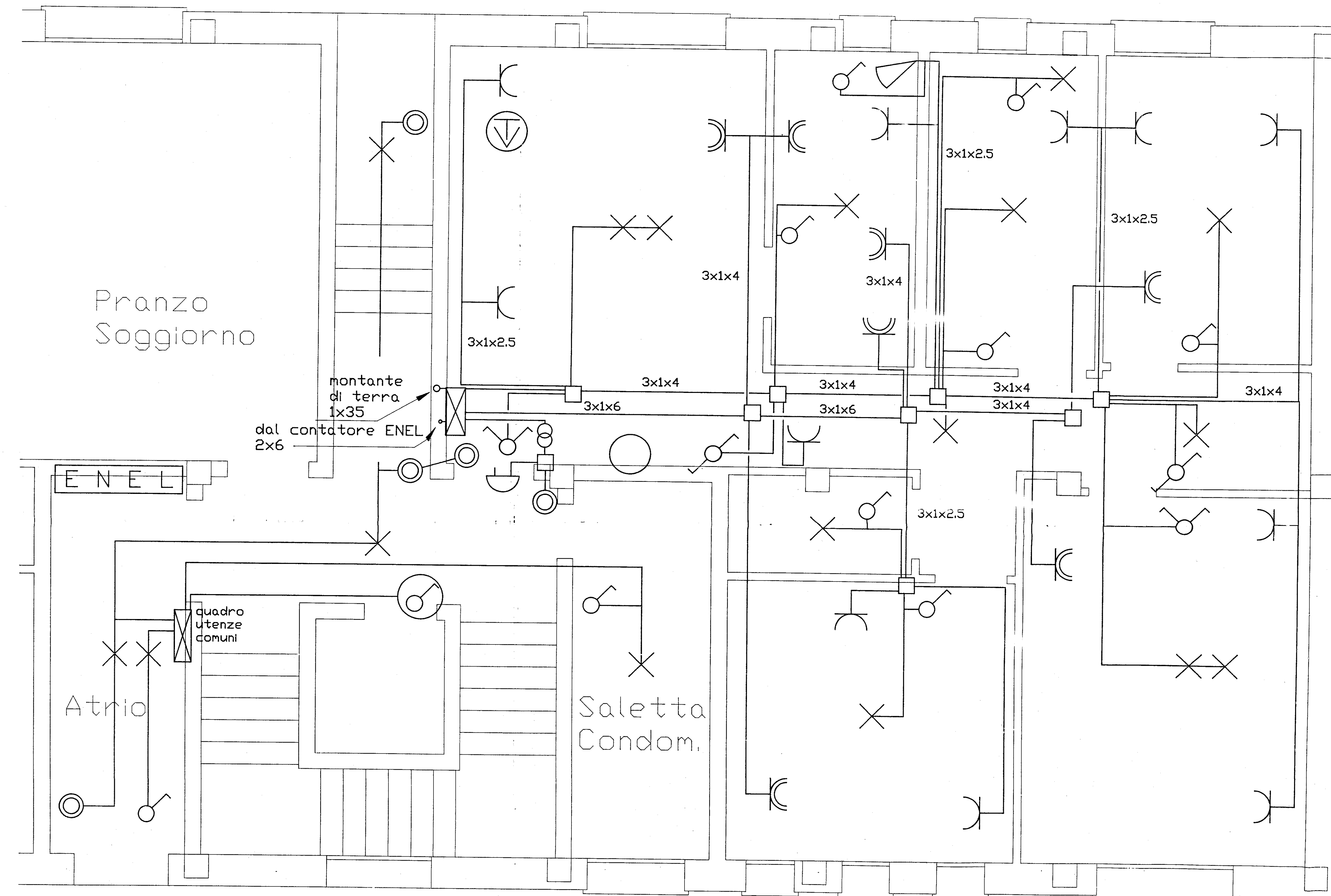
IMPIANTO ELETTRICO PIANO RIALZATO - LOTTO 4 (Scala 1 : 25)
