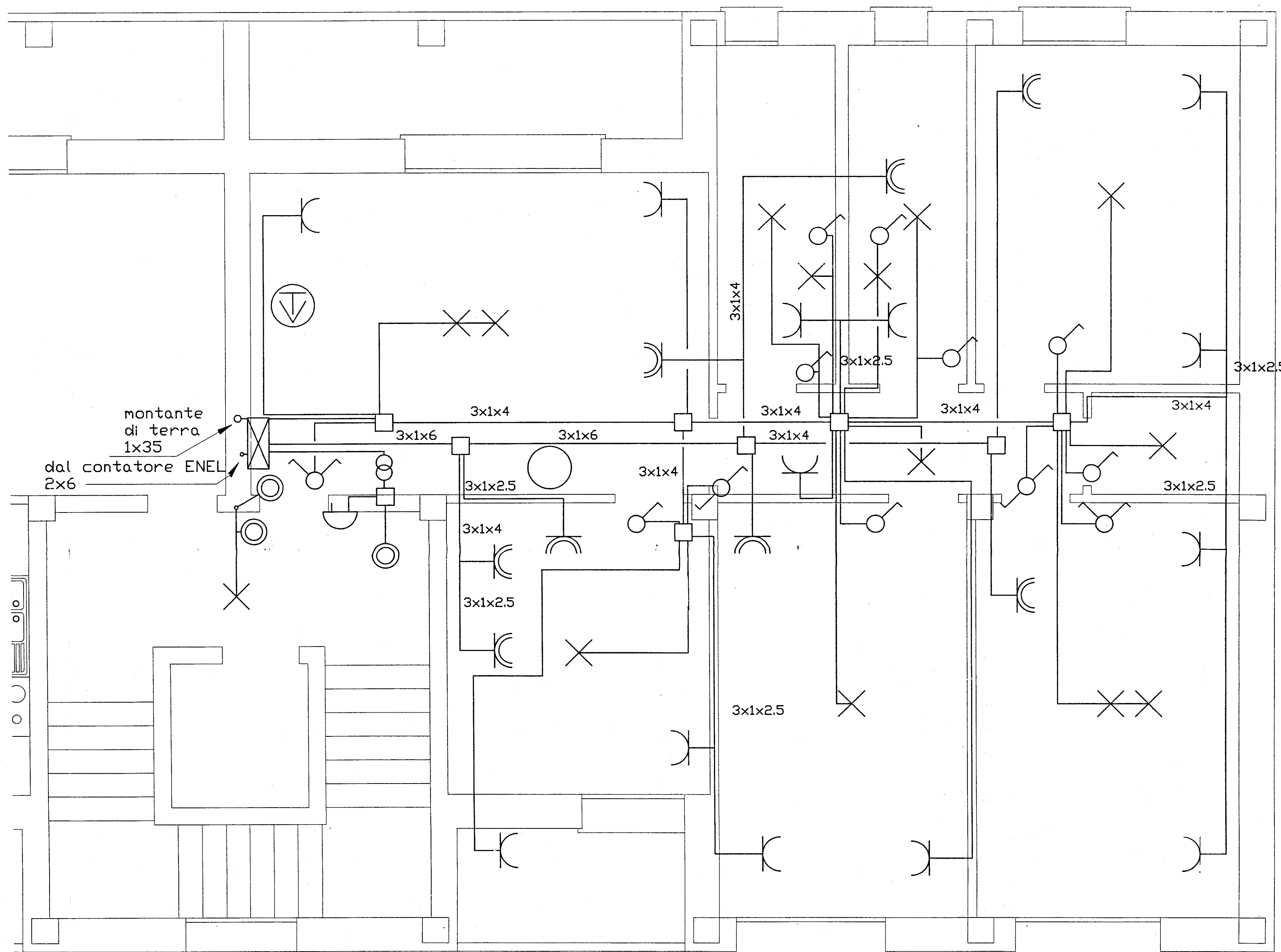
IMPIANTO ELETTRICO PIANO TIPO - LOTTO 4 (Scala 1 : 25)
