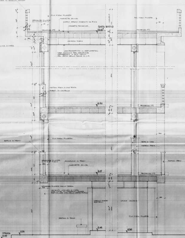
SEZIONE a-b
