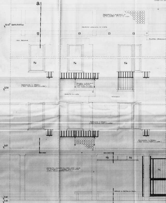
b | PROSPETTO SULL'INGRESSO
