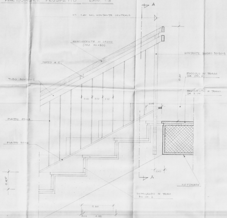
PARTICOLARE PROSPETTO RAPP. 1:5
