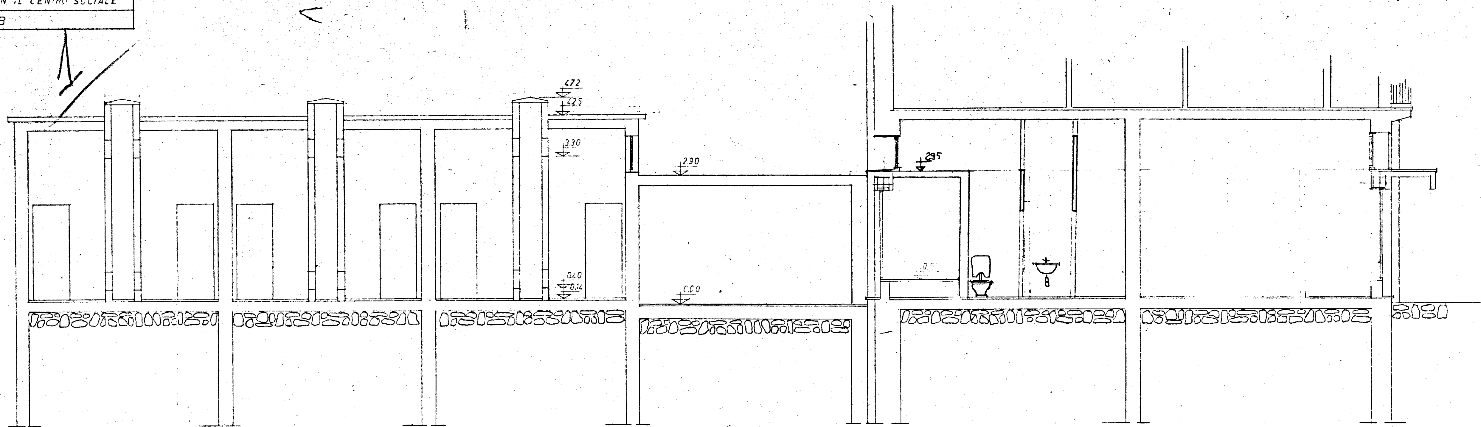
SEZIONE AB
