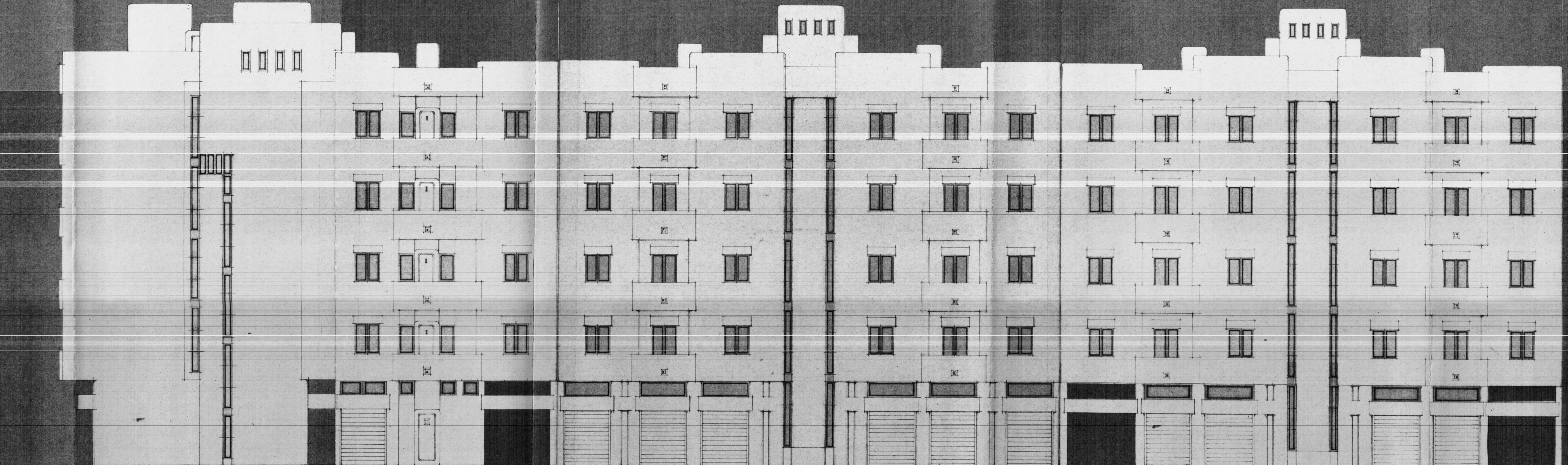
PROSPETTO EST
