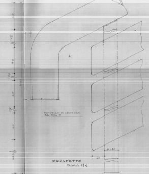
PARTICOLARE COSTRUTTIVO MONTANTE
