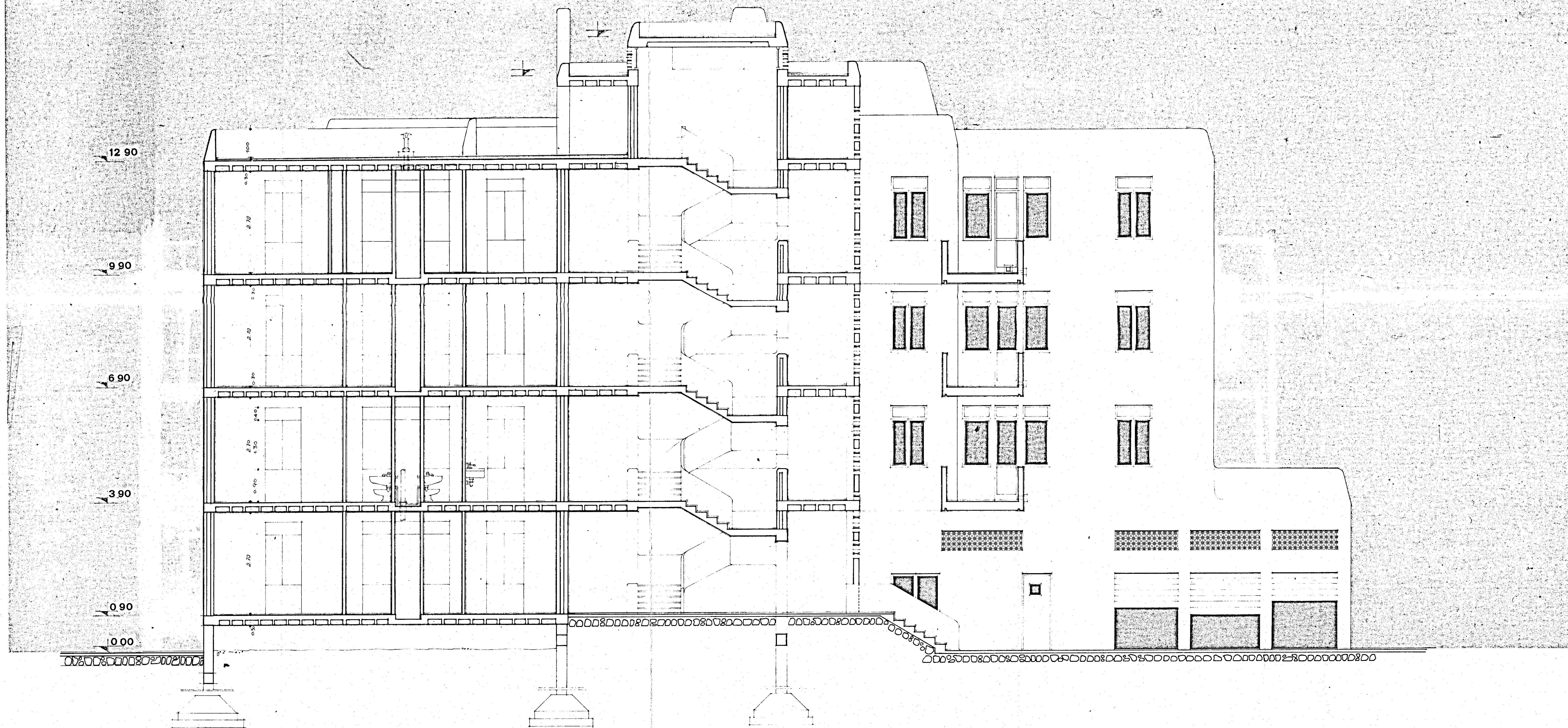
SEZIONE A-A'
