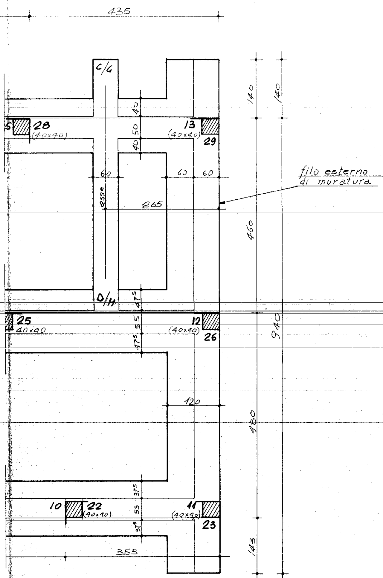
VARIANTE DI TESTATA PER LE PALAZZINE ACCOPIATE
