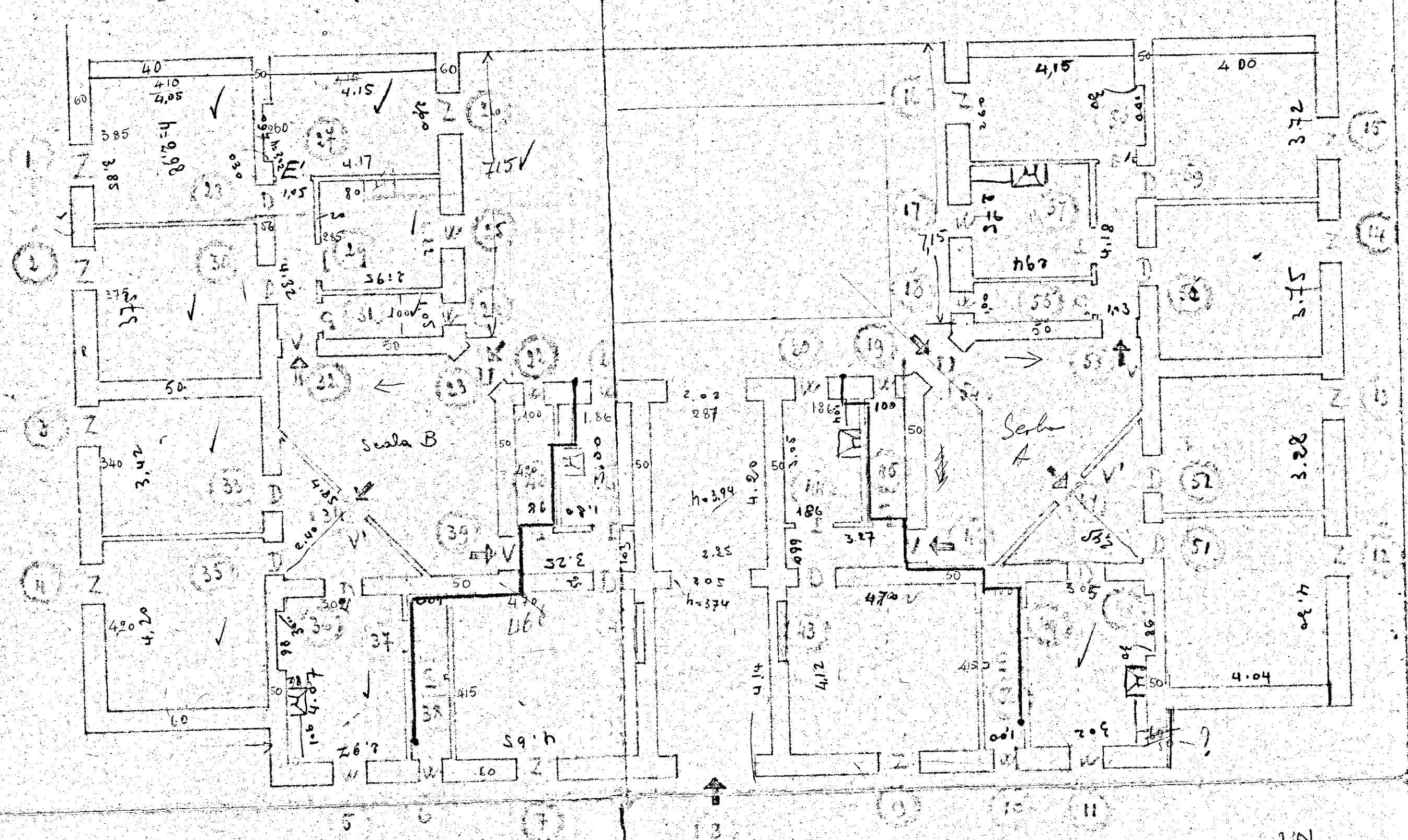
- II° LOTTO - PIANTA PIANO TERRENO -
