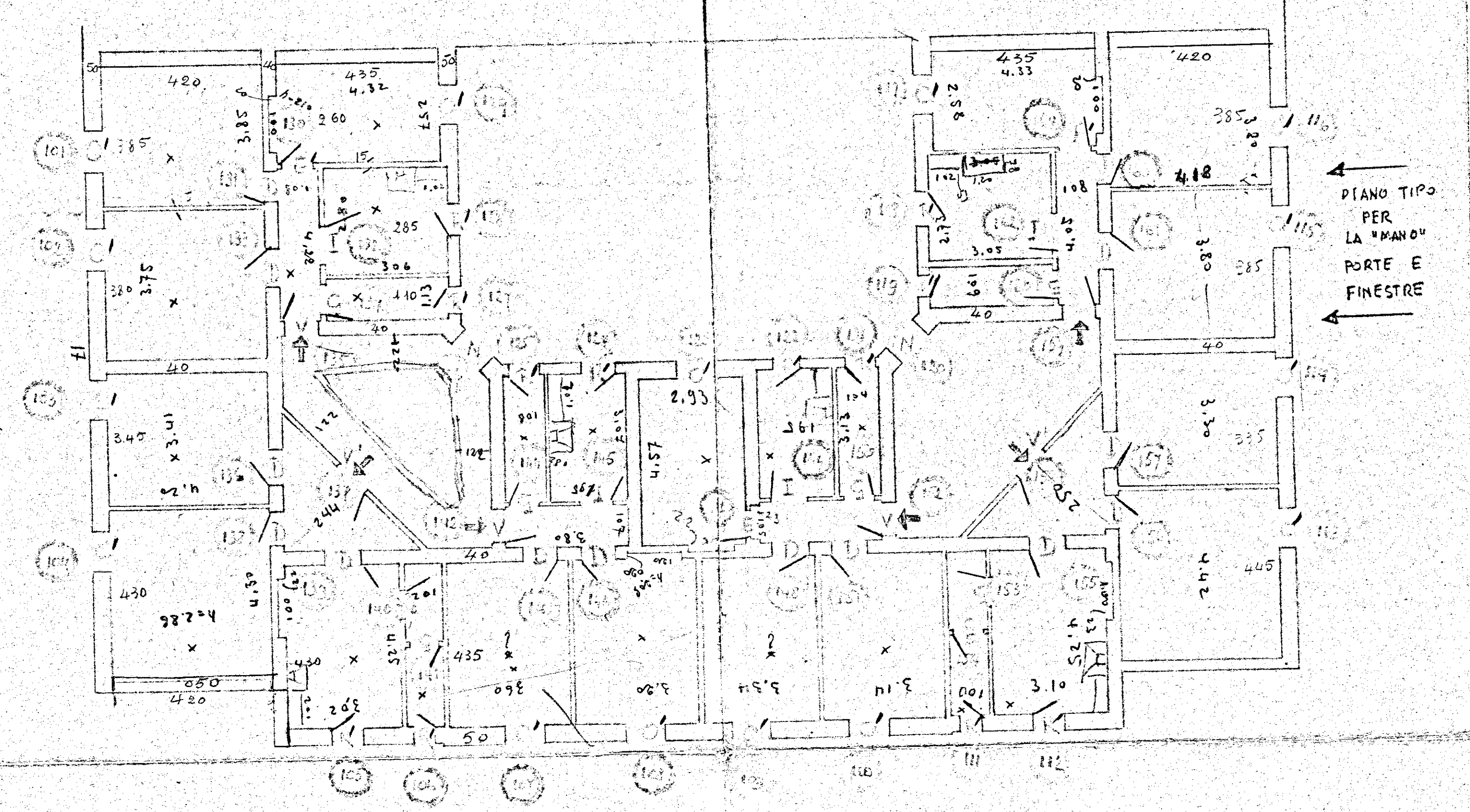
II° LOTTO - PIANTA I° PIANO -
