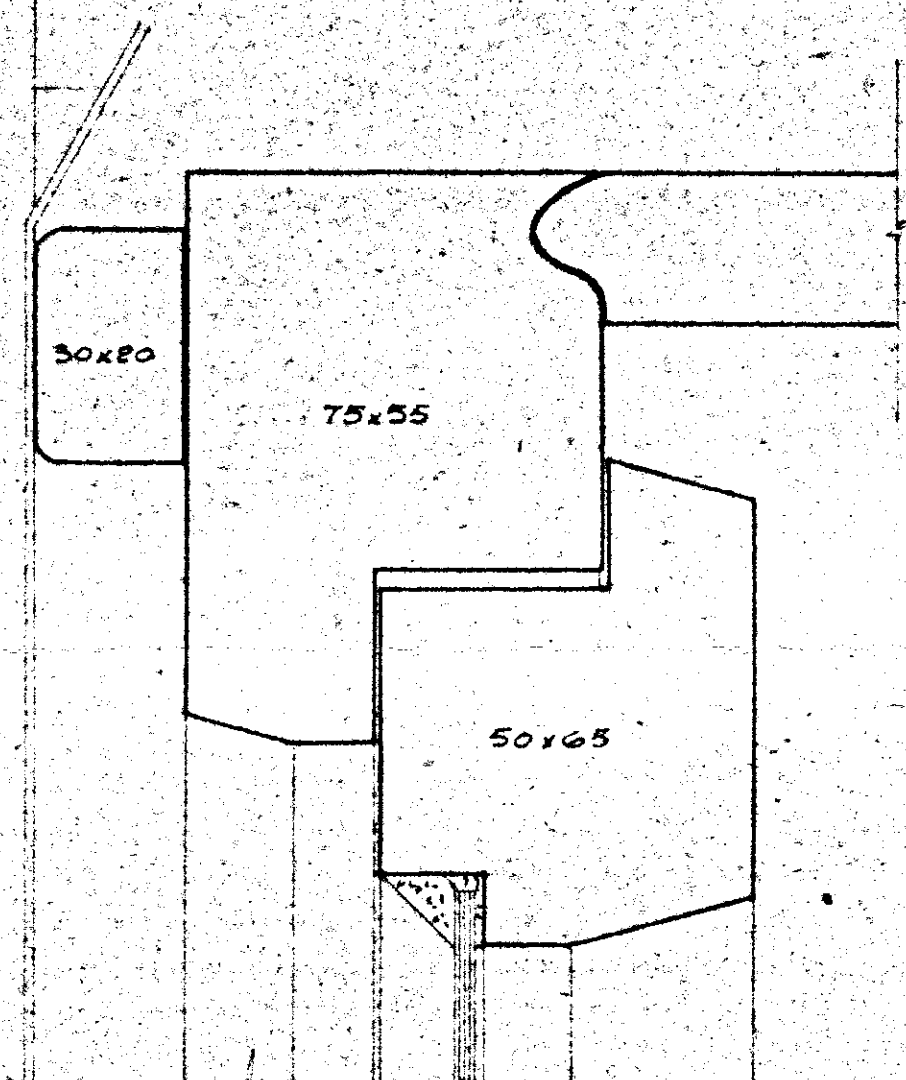
SEZIONE 1 TAV. 19
