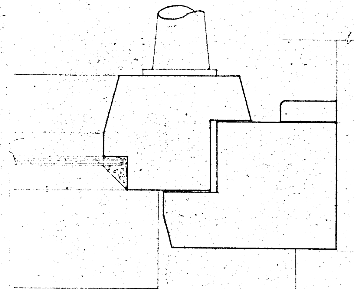
SEZIONE 5 TAV. 19
