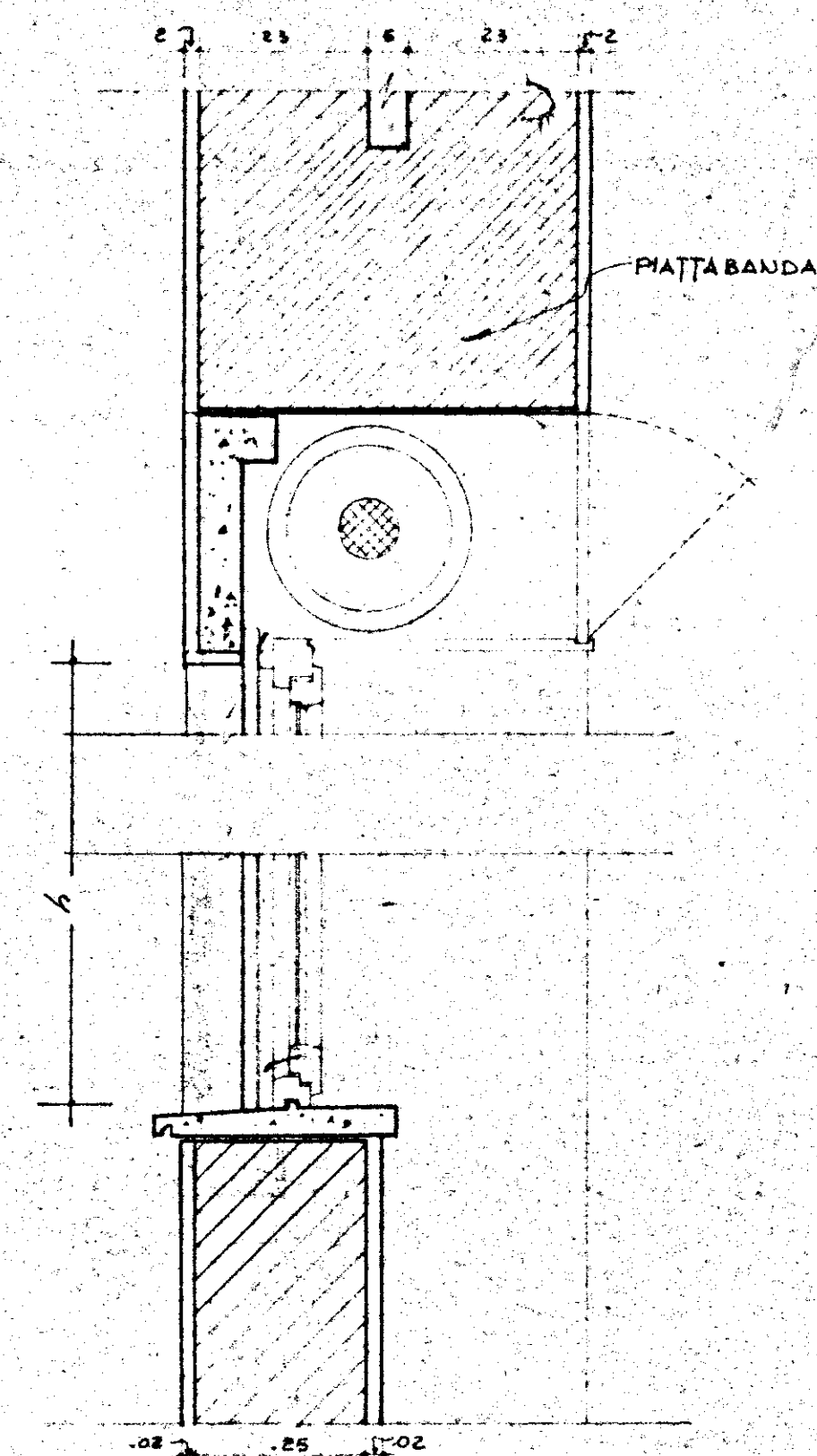
SEZIONE TIPO VERT.
