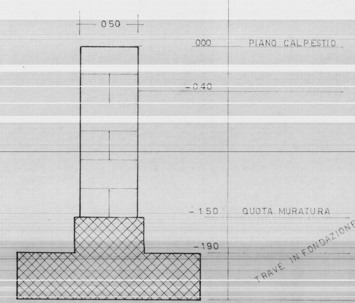
SEZIONE MURATURA
