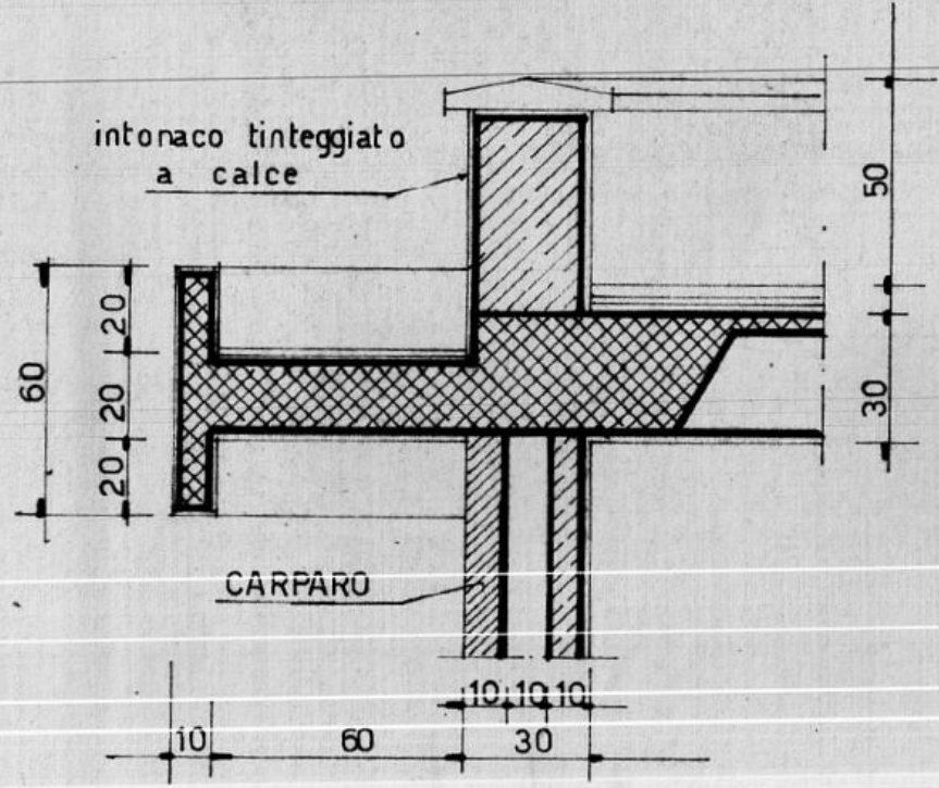
particolare A B rapp. 1:20
