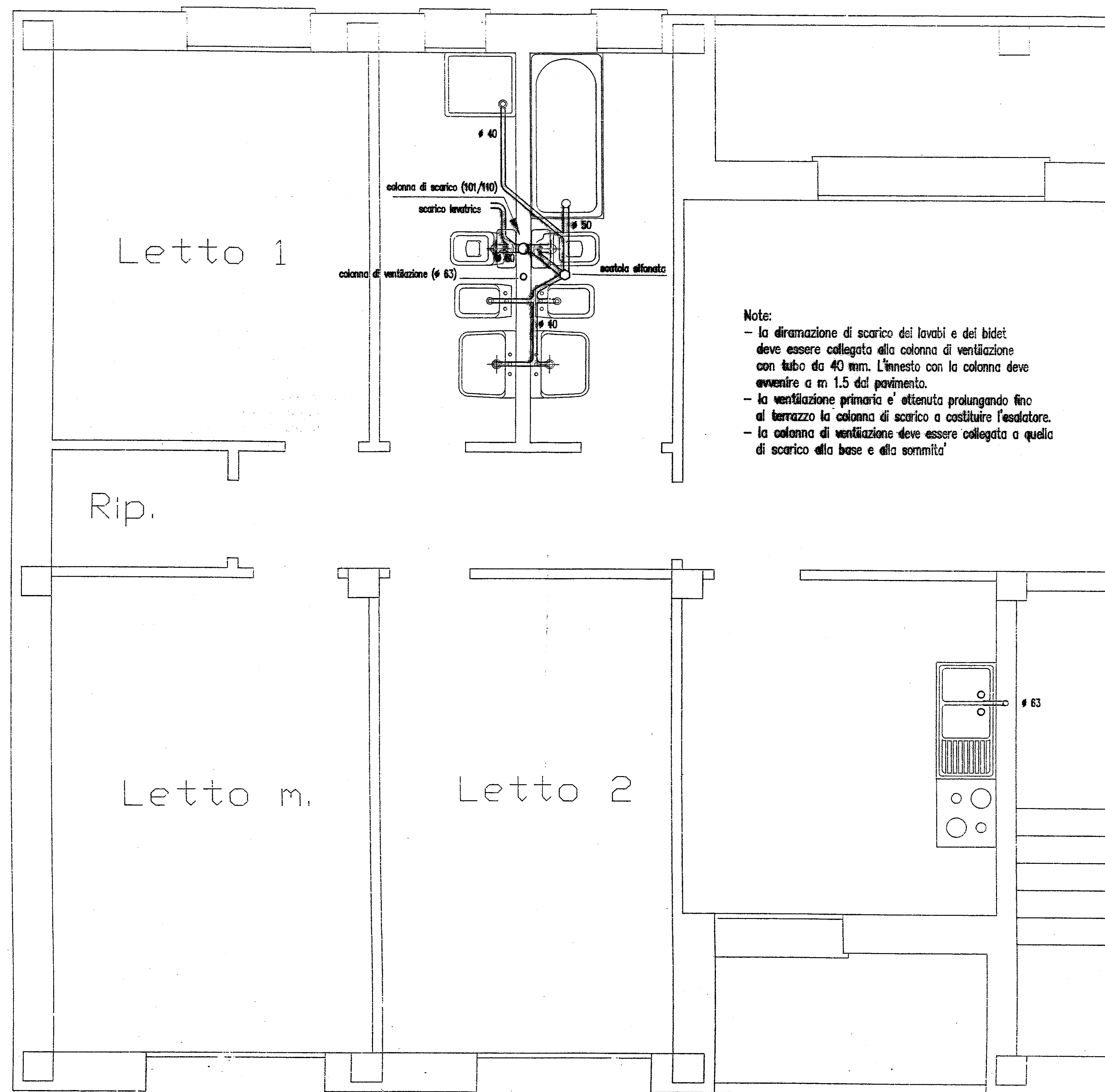
RETE DI SCARICO APPARTAMENTO TIPO - LOTTO 3 (Scala 1 : 25)
