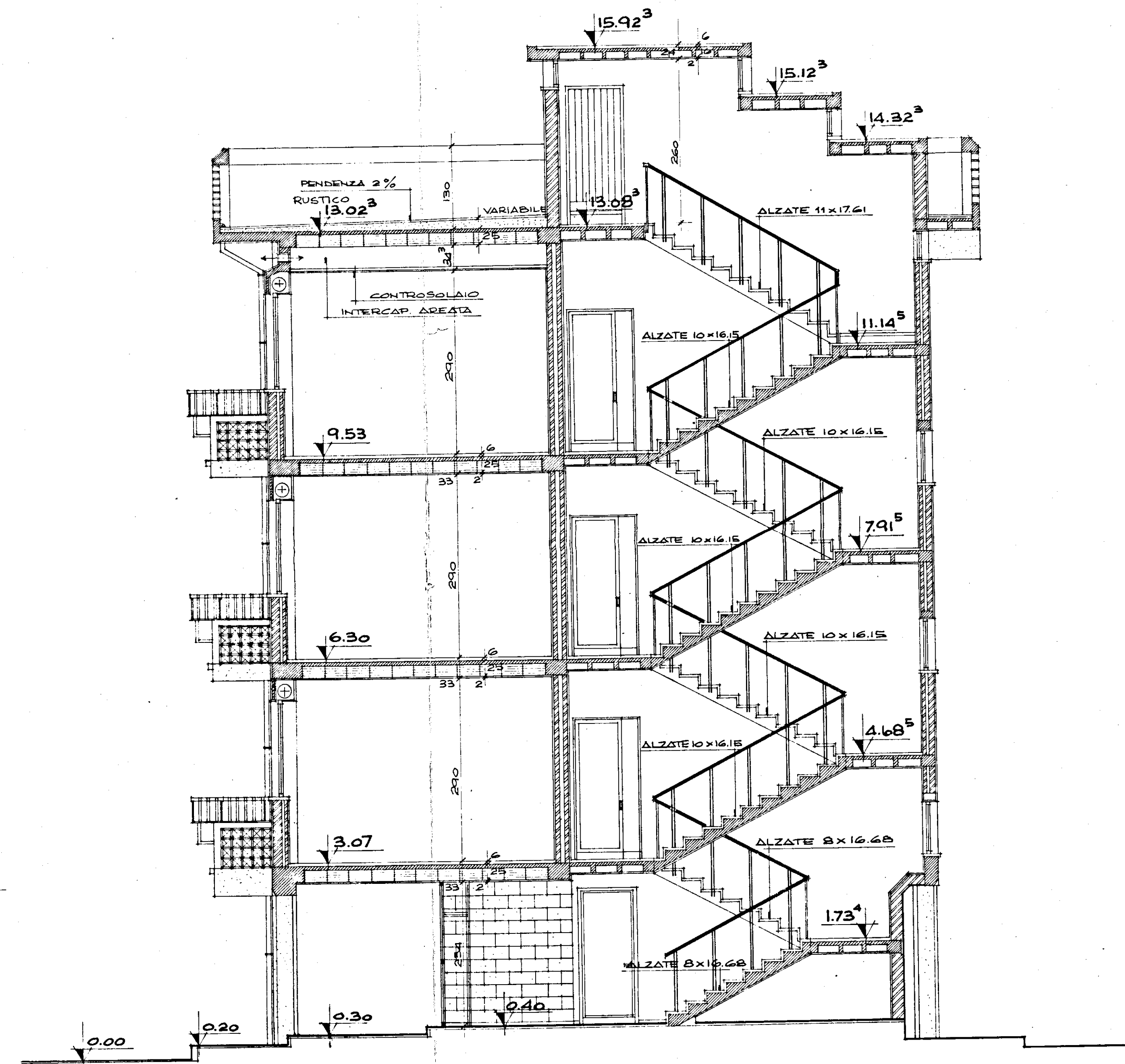
SEZIONE a-b
