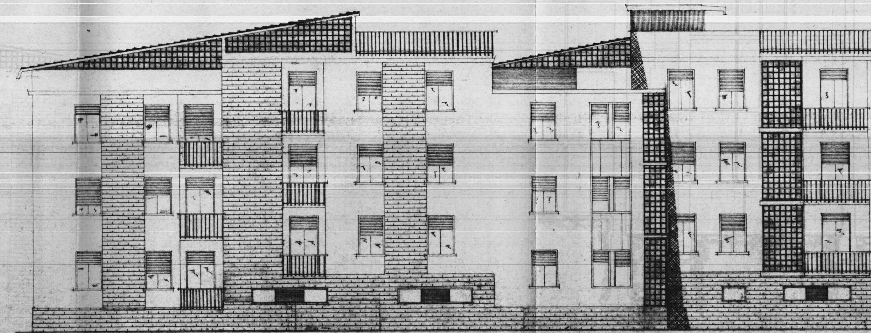
PROSPETTO POSTERIORE
