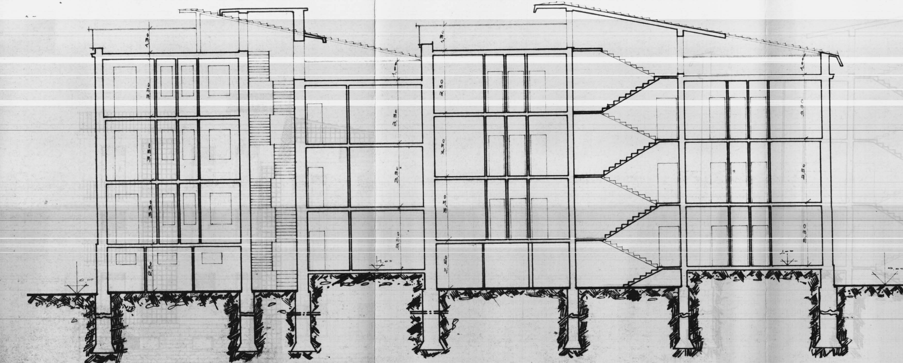
SEZIONE LONGITUDINALE
