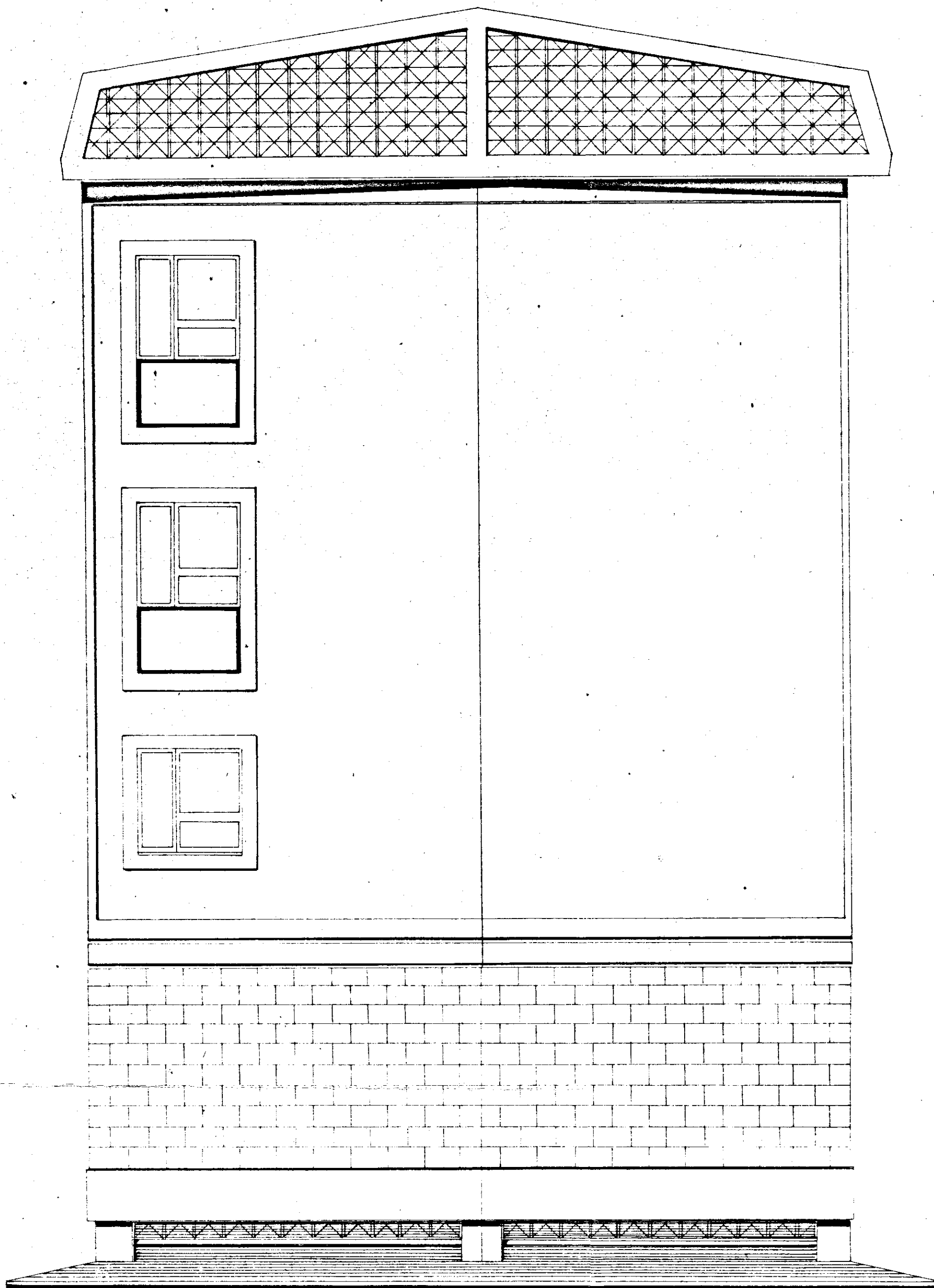
FRONTE TERMINALE scala 1 : 50
