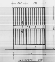
PROSPETTO 1:20
