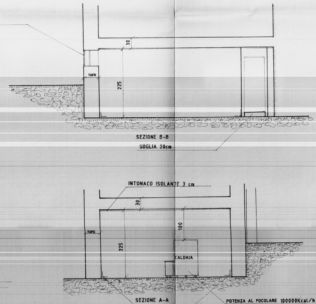
SEZIONE A-A
