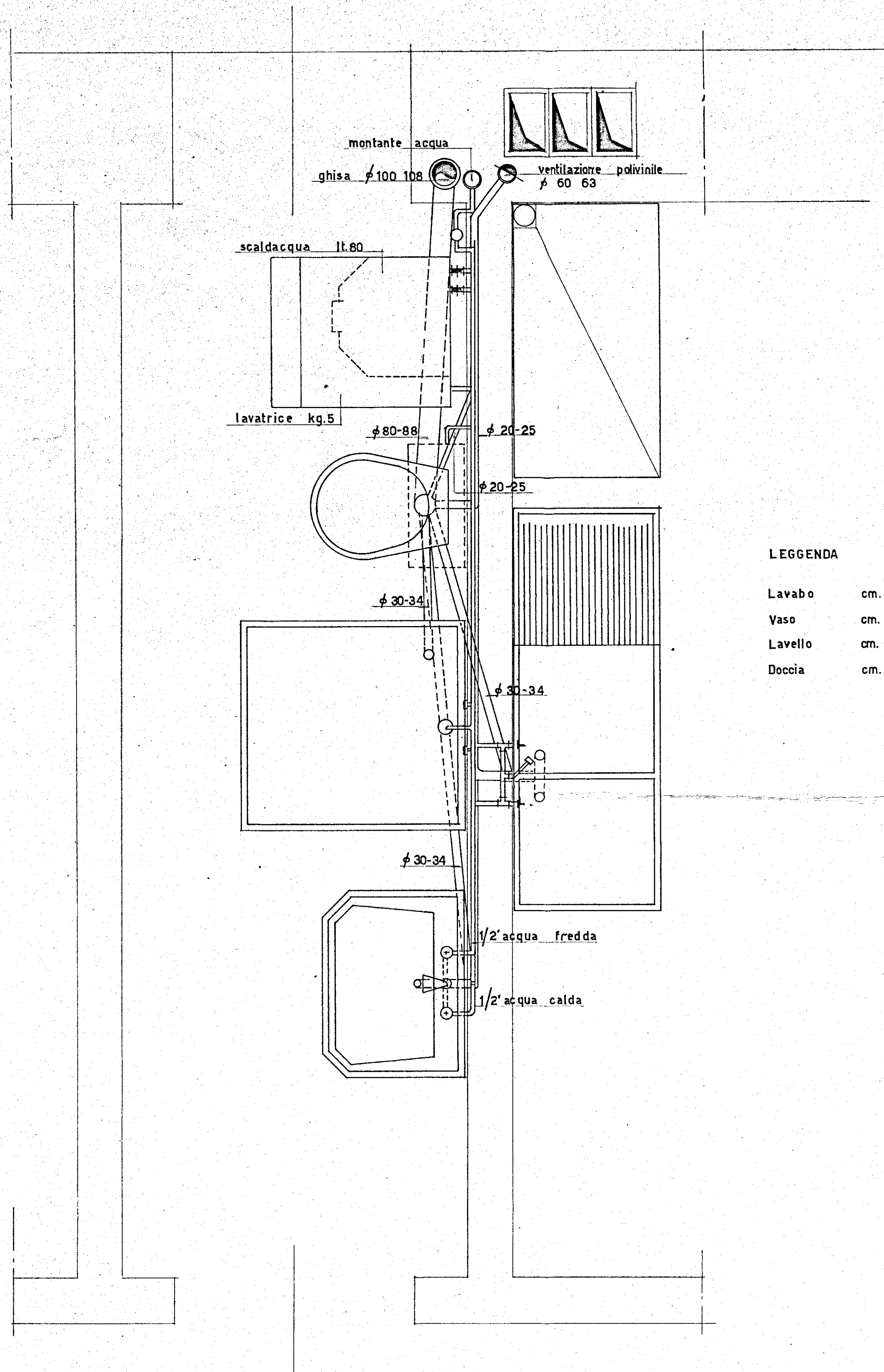
PIANTA Rapp. 1:10
