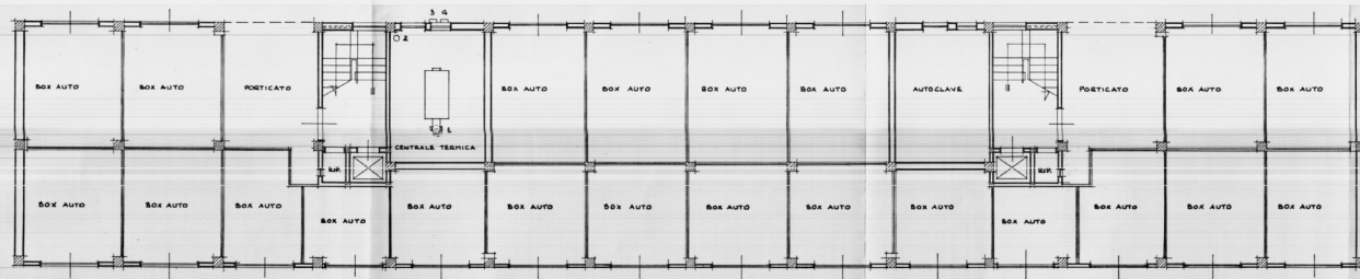
PIANTA PIANO TERRENO
