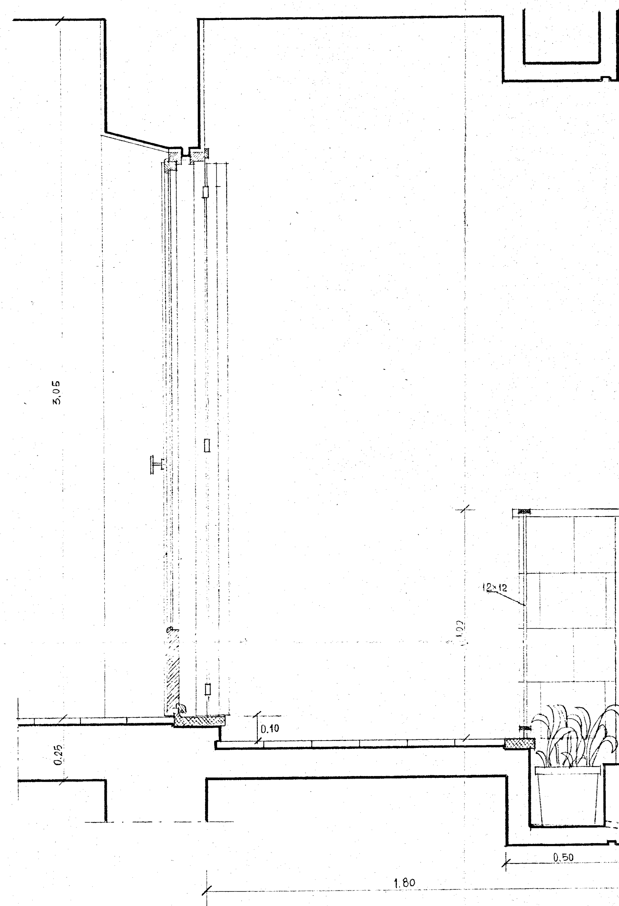
SEZIONE A-B
