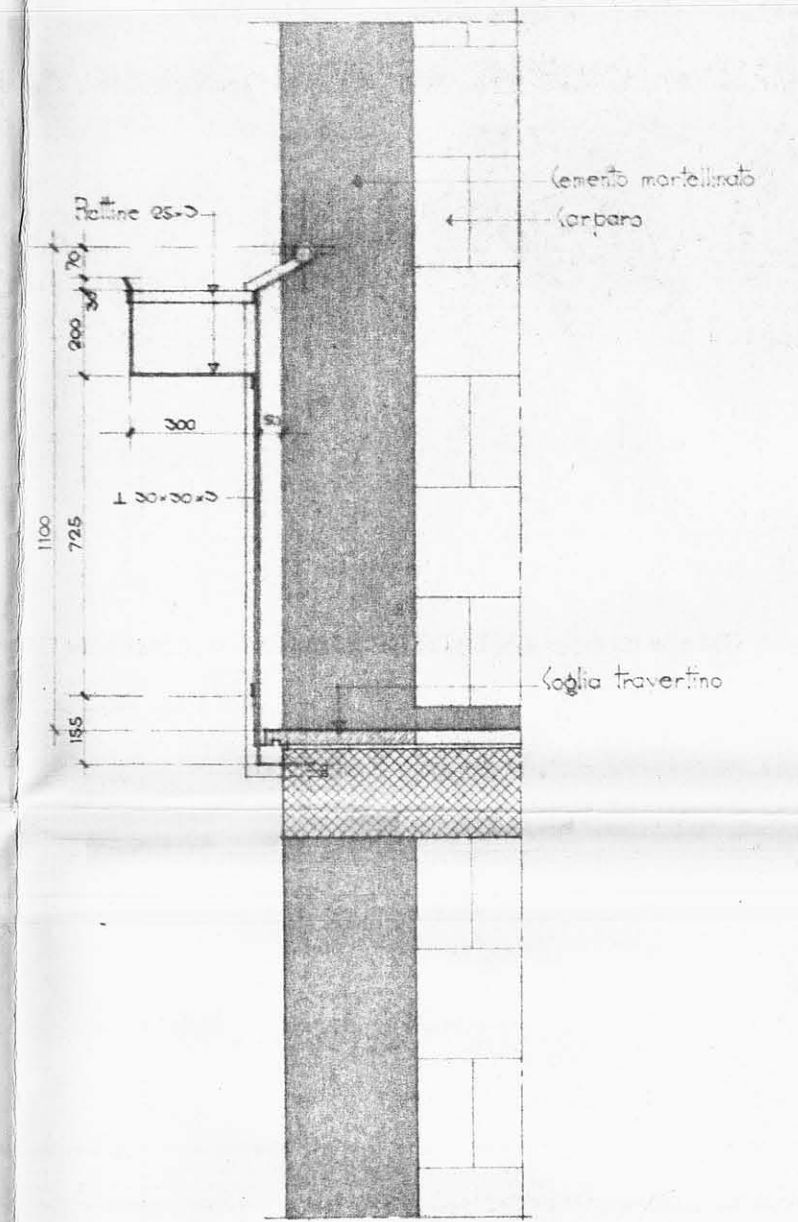
SEZIONE
