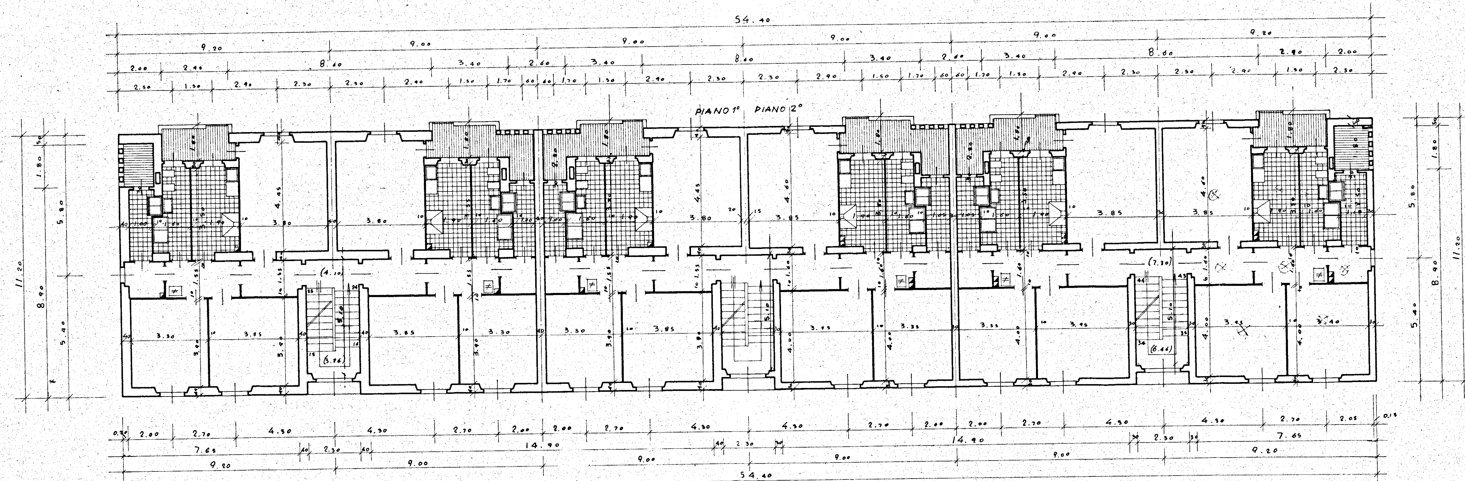
DIS. 57 PIANTE PIANI 1° E 2° RAPP. 1:100
