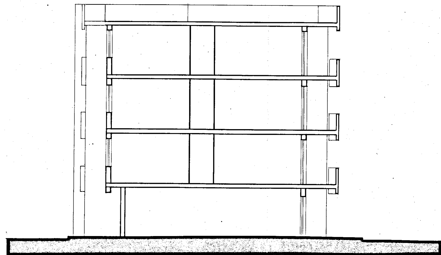
sez aa
