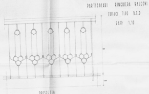
PARTICOLARI RINGHIERA EDIFICI TIPO B.C. RAPP. 1:10
