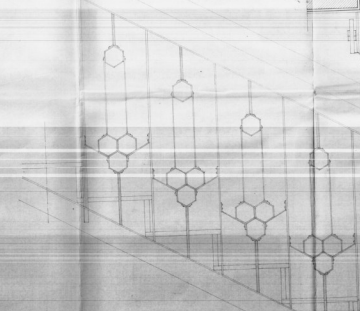
PARTICOLARI SCALE E RINGHIERA EDIFICI TIPO B.C.D. RAPP. 1:10
