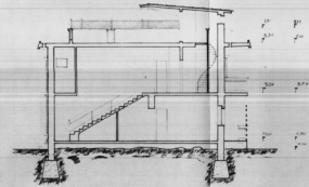
SEZIONE A-A
