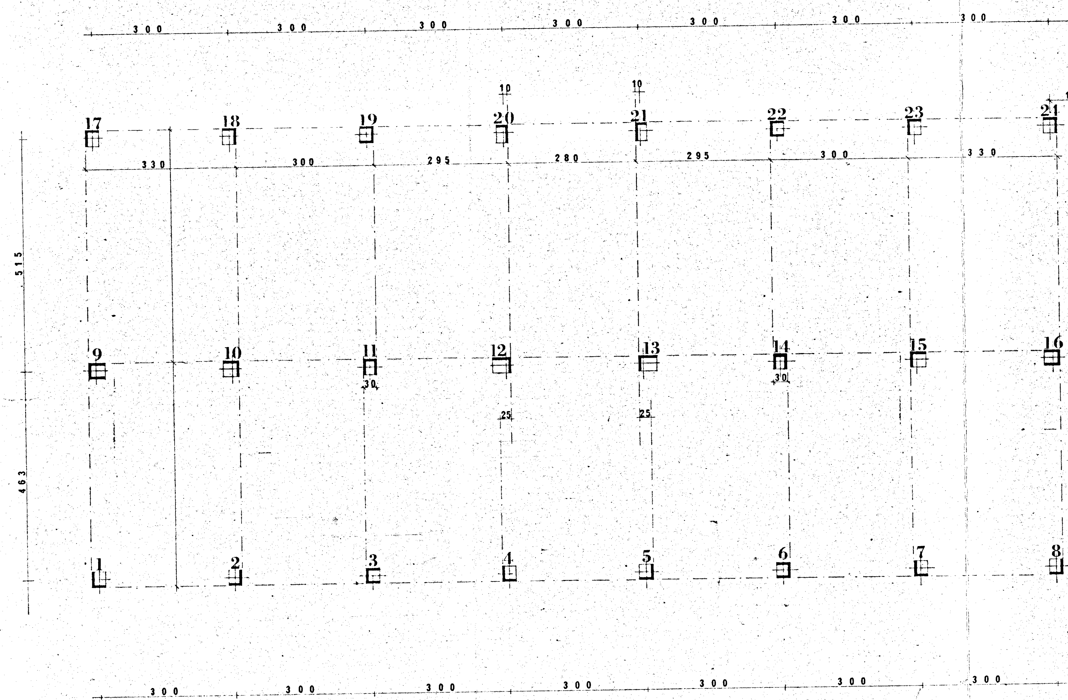
PIANTA DEI FILI DEI PILASTRI rapp. 1:50
