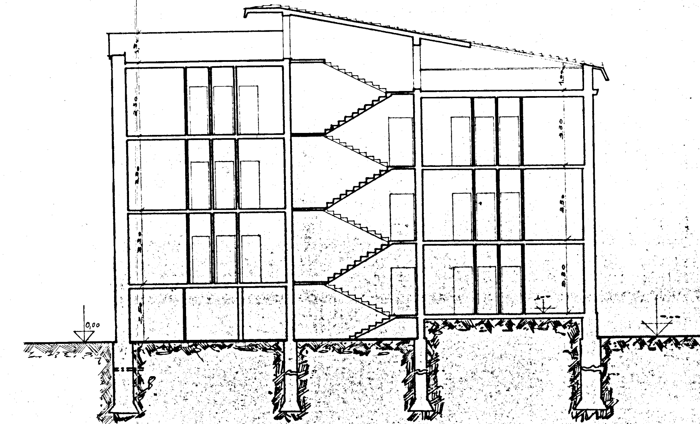
SEZIONE LONGITUDINALE
