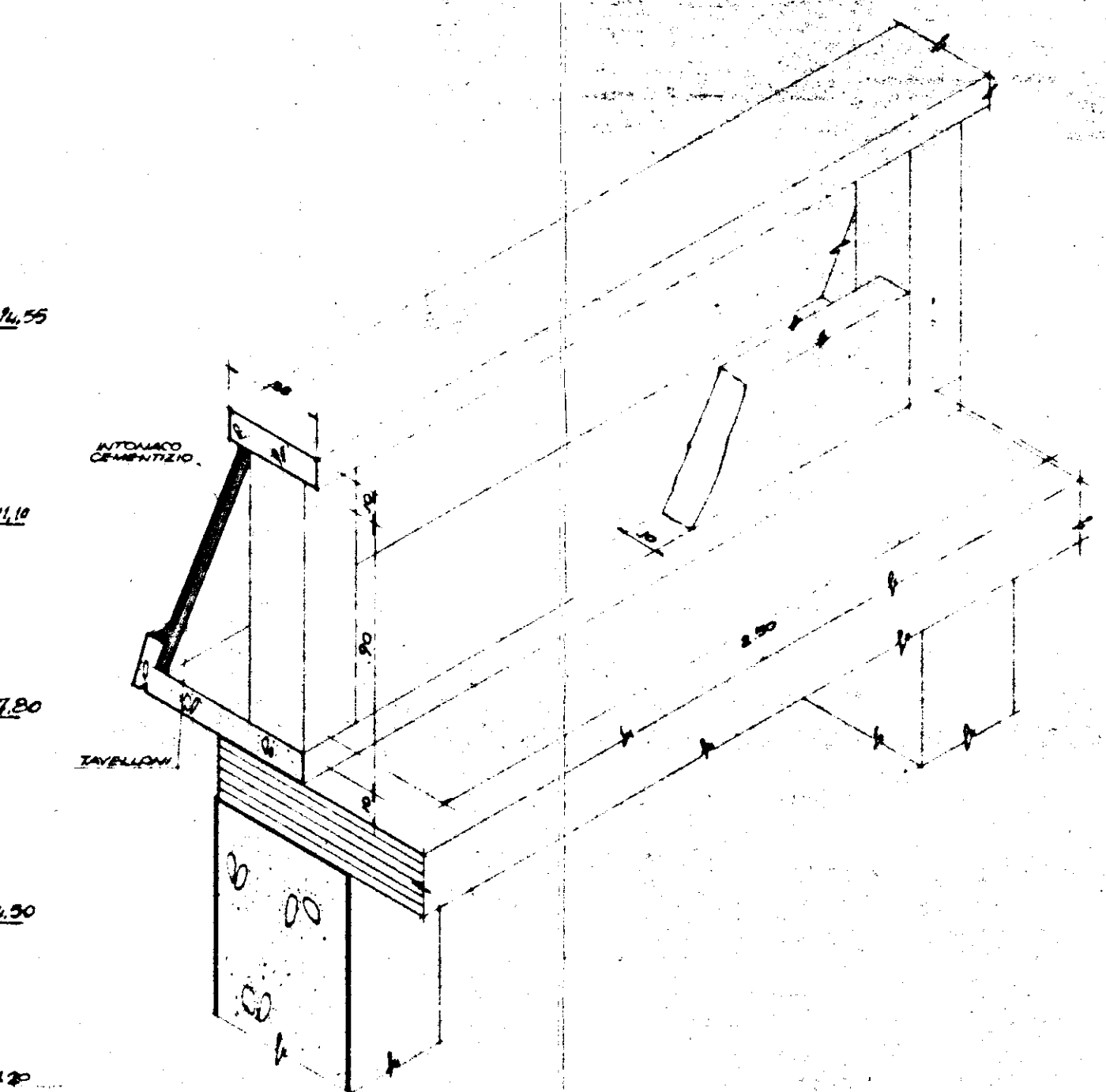
NODO 'A. VISTA ASSONOMETRICA
