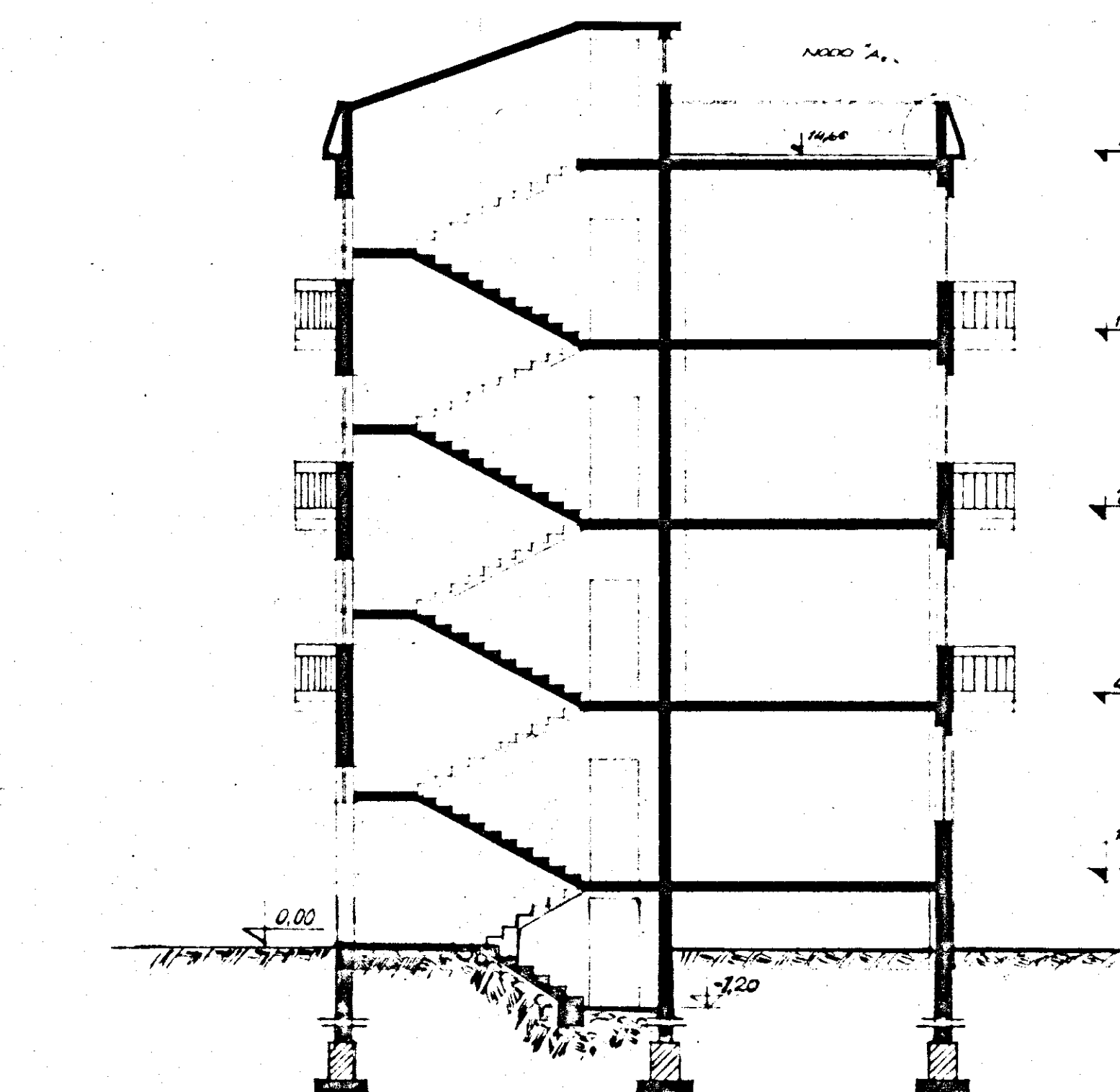
SEZIONE X-X
