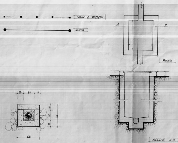
PARTICOLARE ATTRAVERSAMENTO
