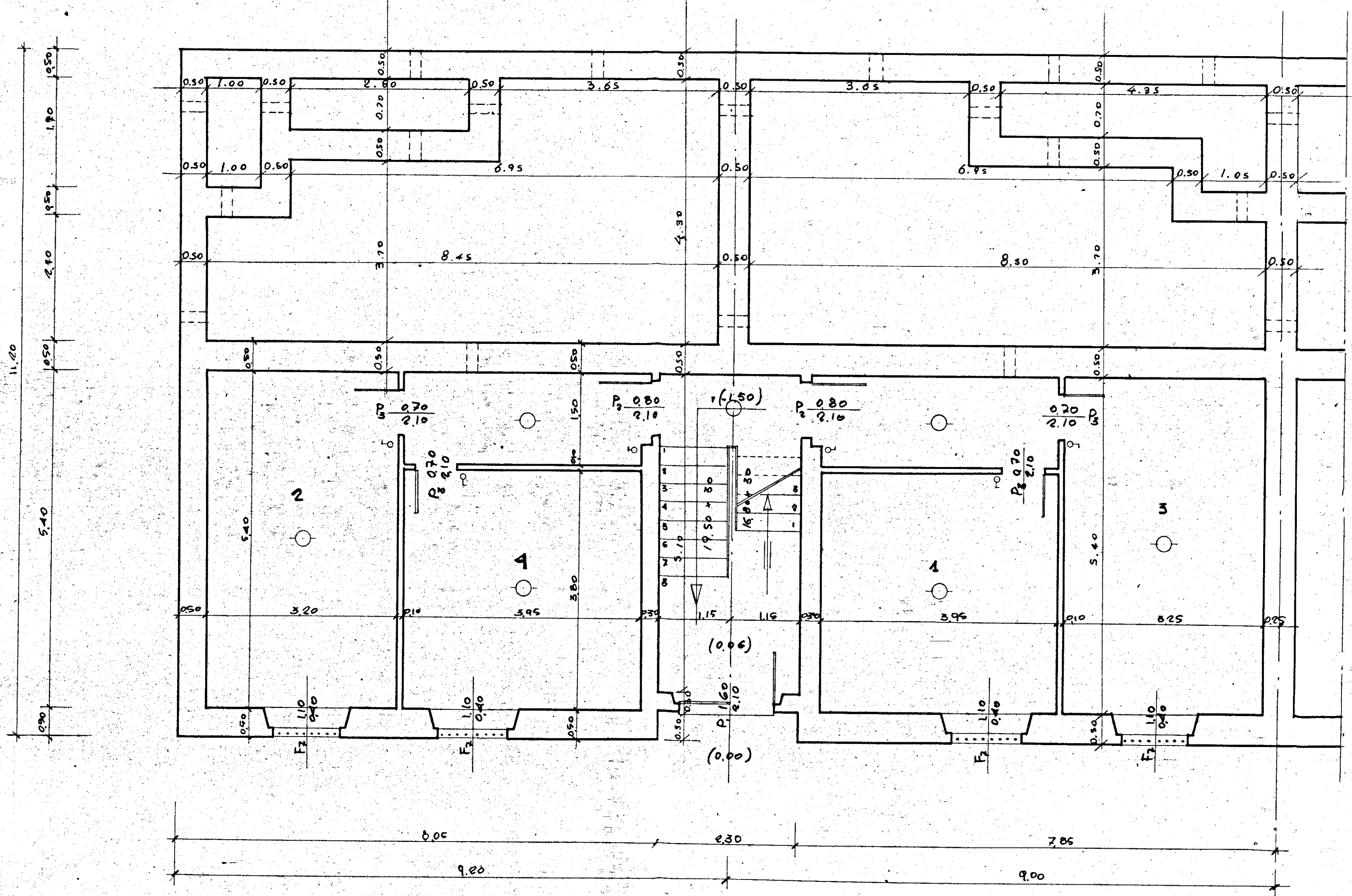
DIS. 140 bis PARTICOLARE PIANTE CANTINE RAPP. 1:50
