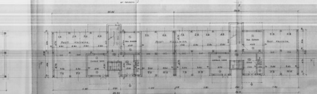
PIANTA PIANO TERRA
