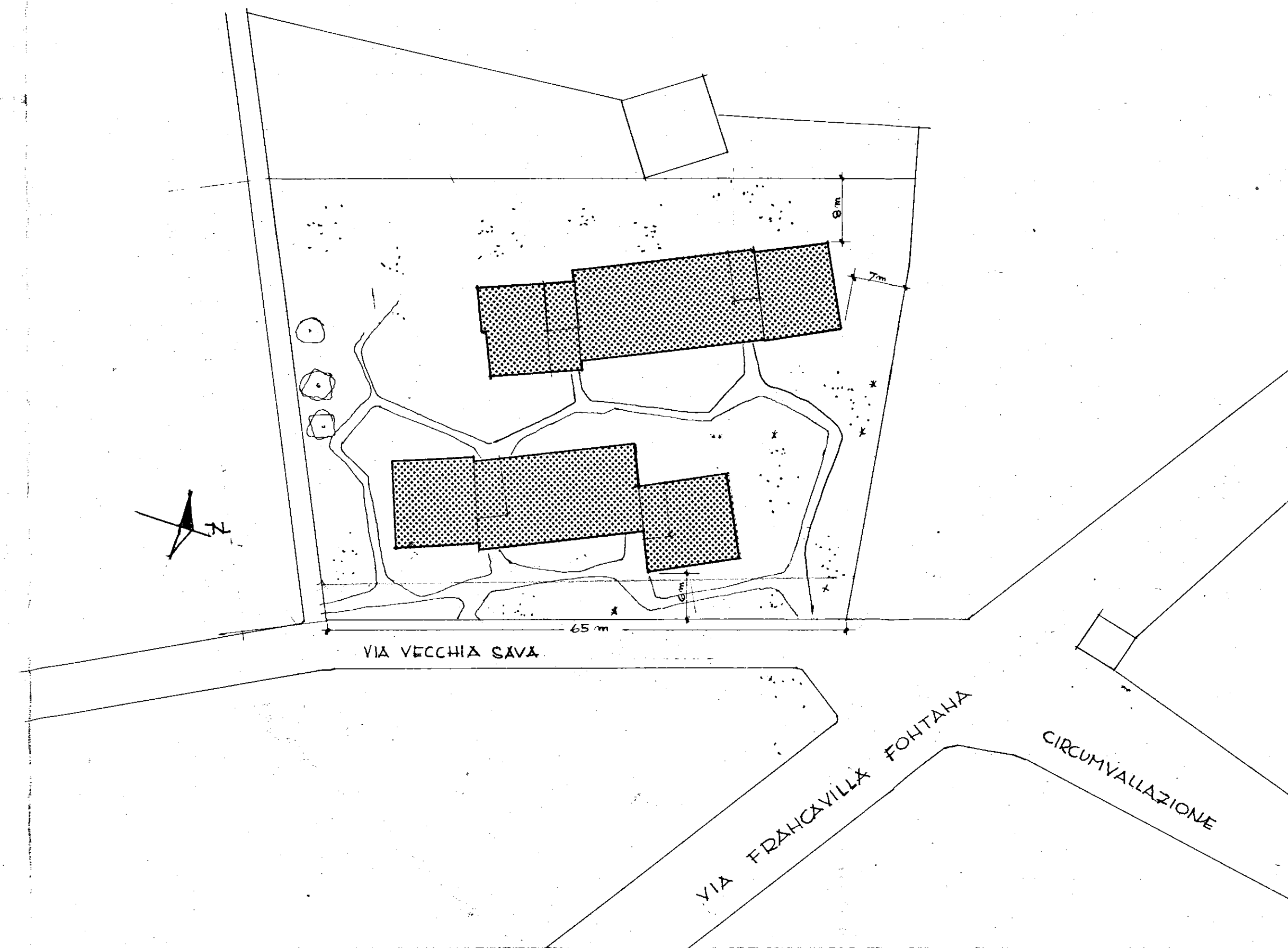
PLANIMETRIA GENERALE 1:500
