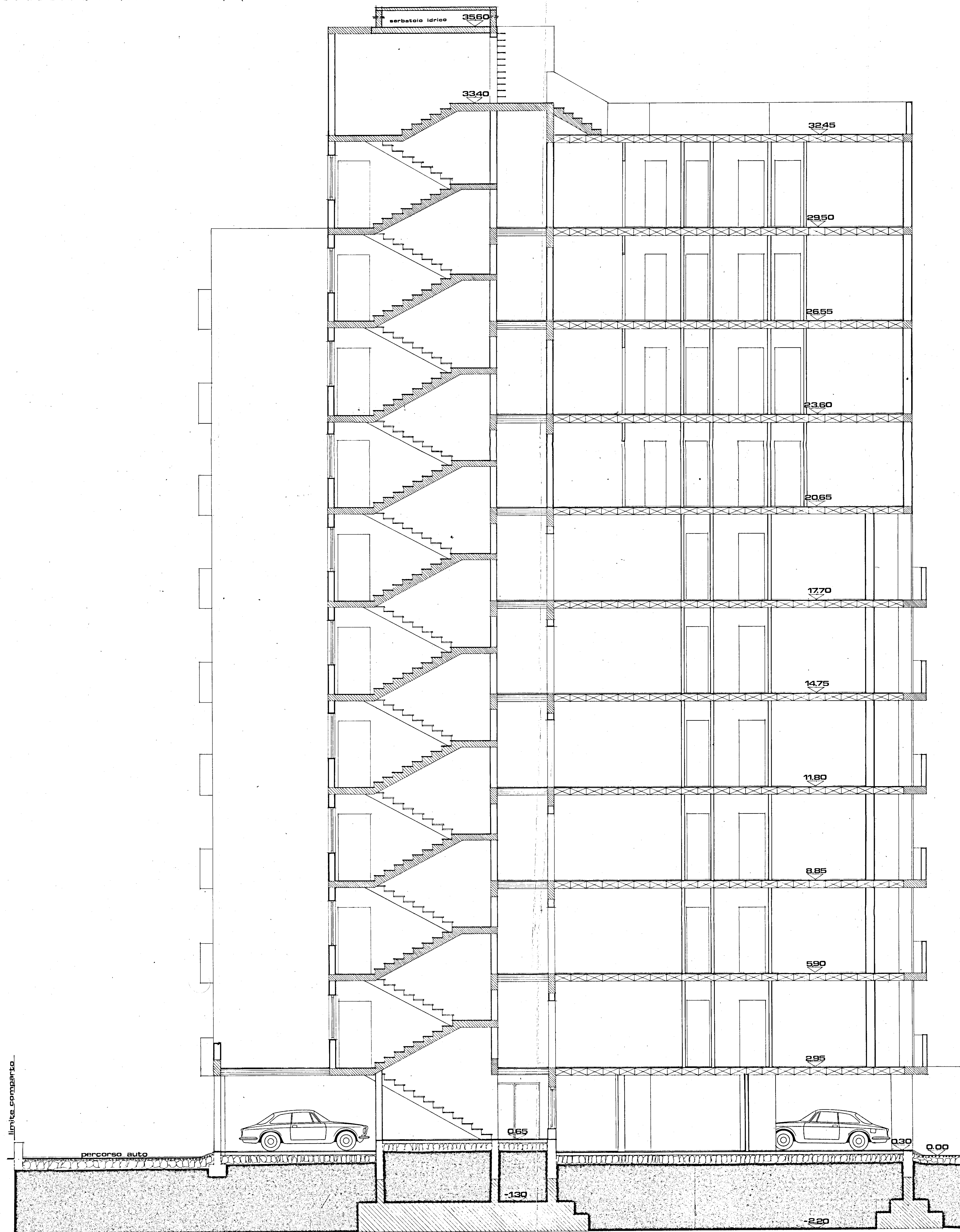
SEZIONE B-B
