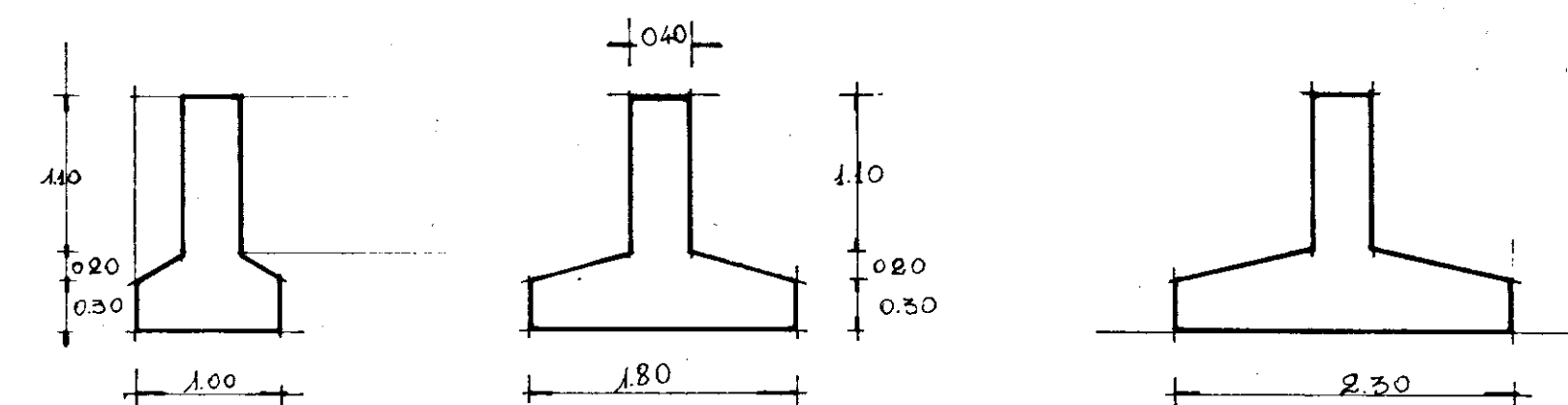
Sezione A-B
