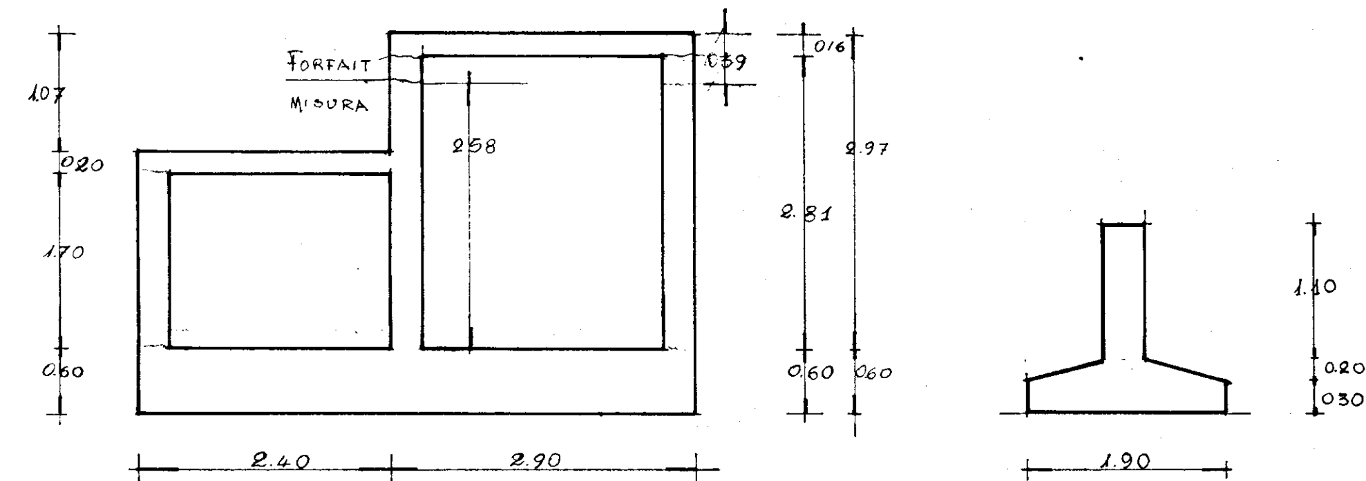
Sezione G-H
