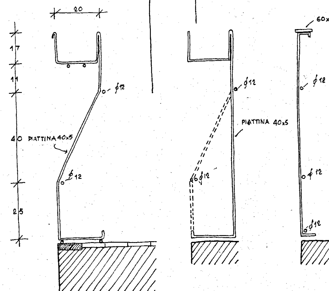
SEZIONE C-D
