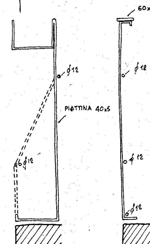
SEZIONE C-D
