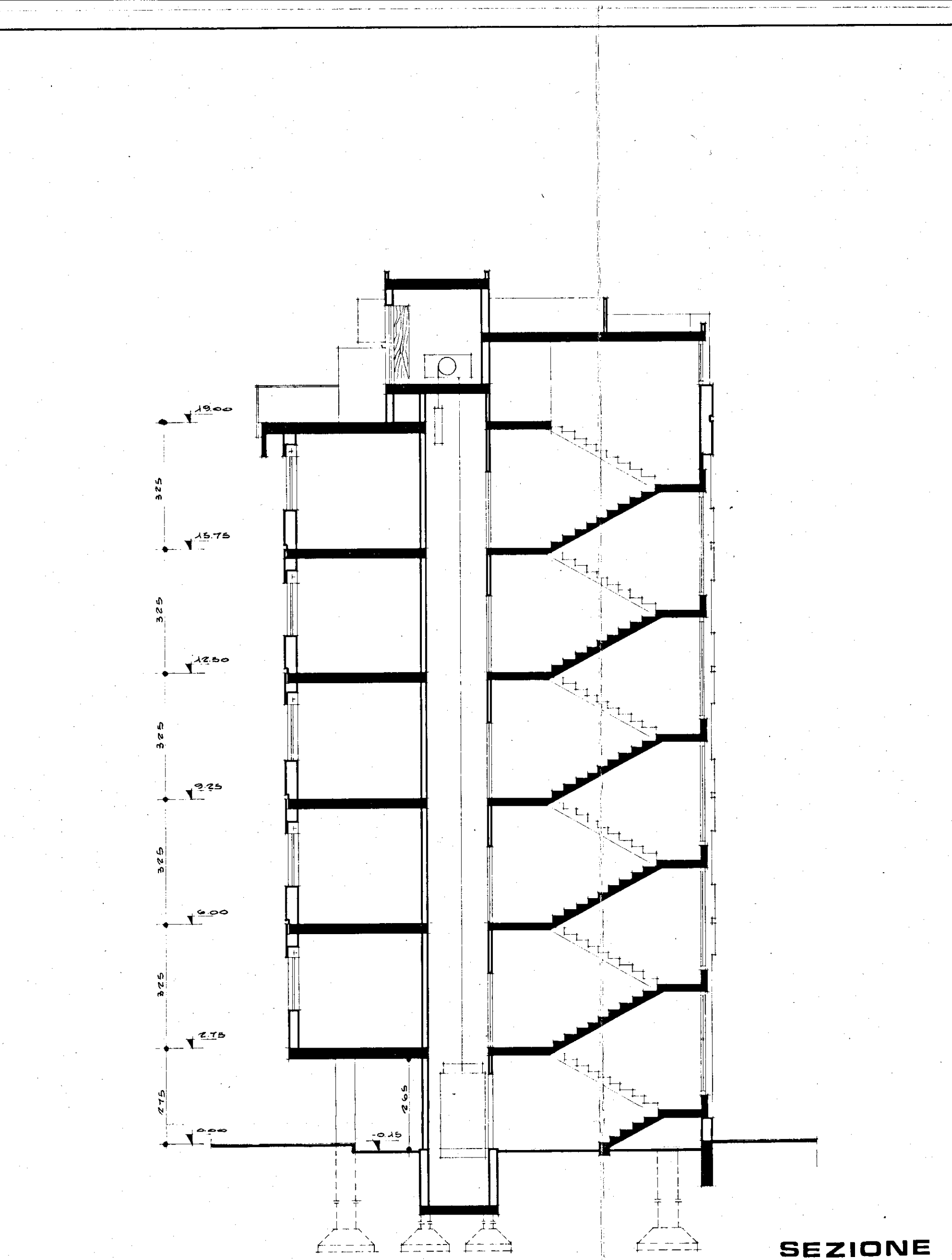
SEZIONE A-A
