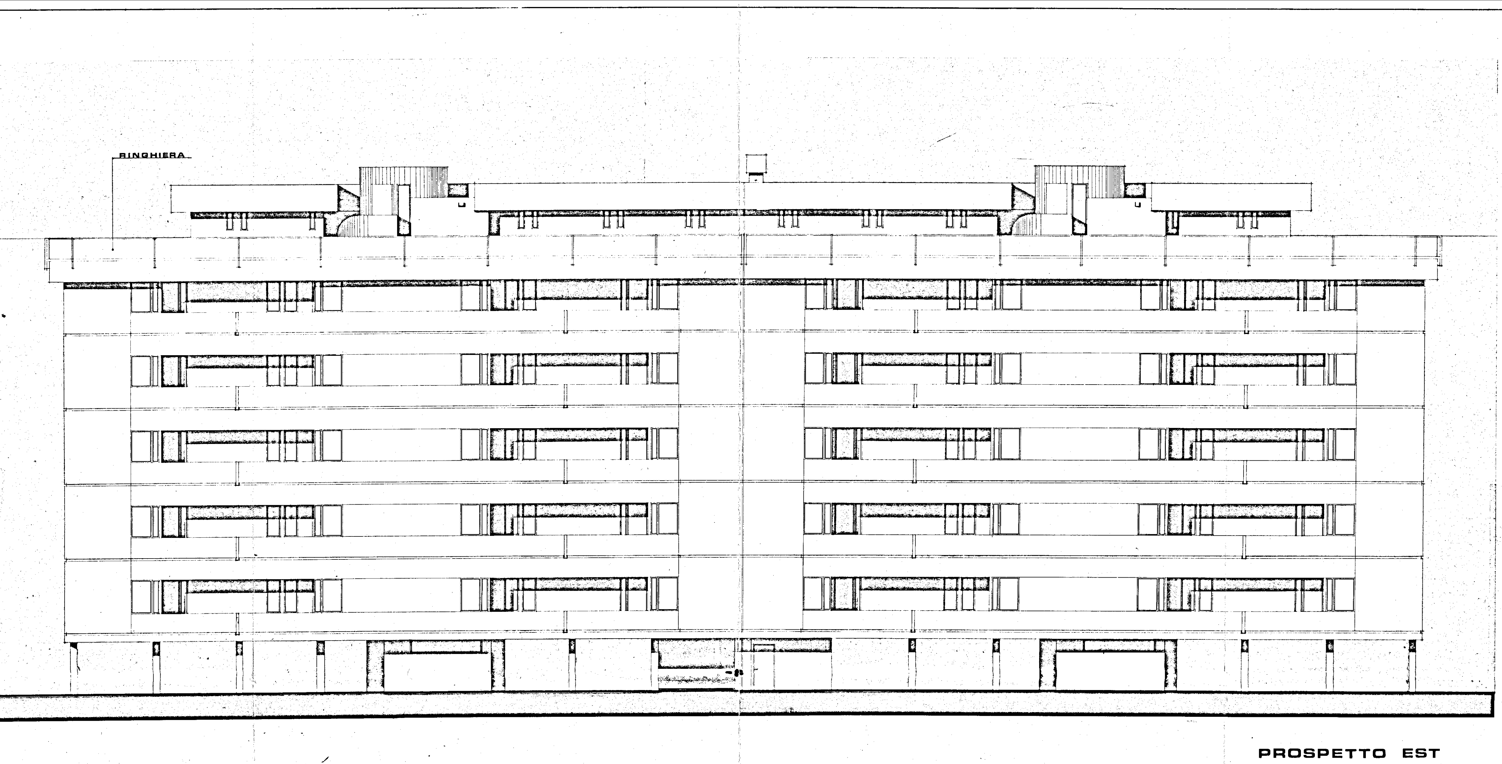
PROSPETTO EST
