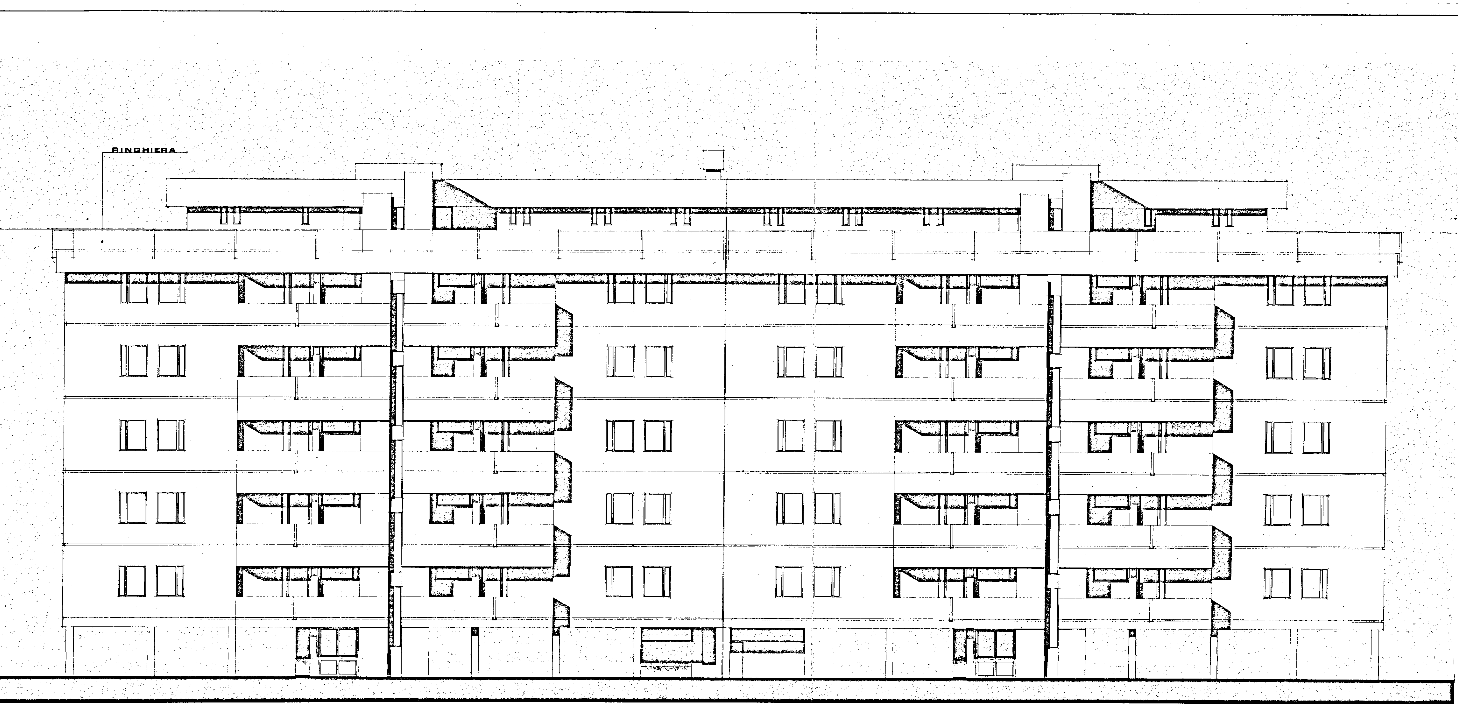
PROSPETTO OVEST
