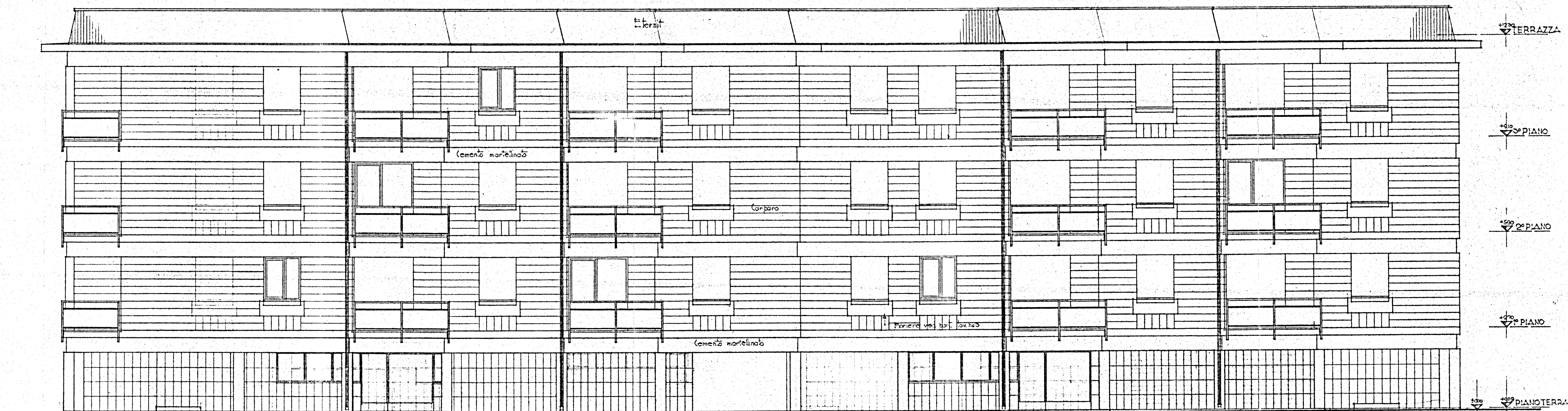
PROSPETTO A-B
