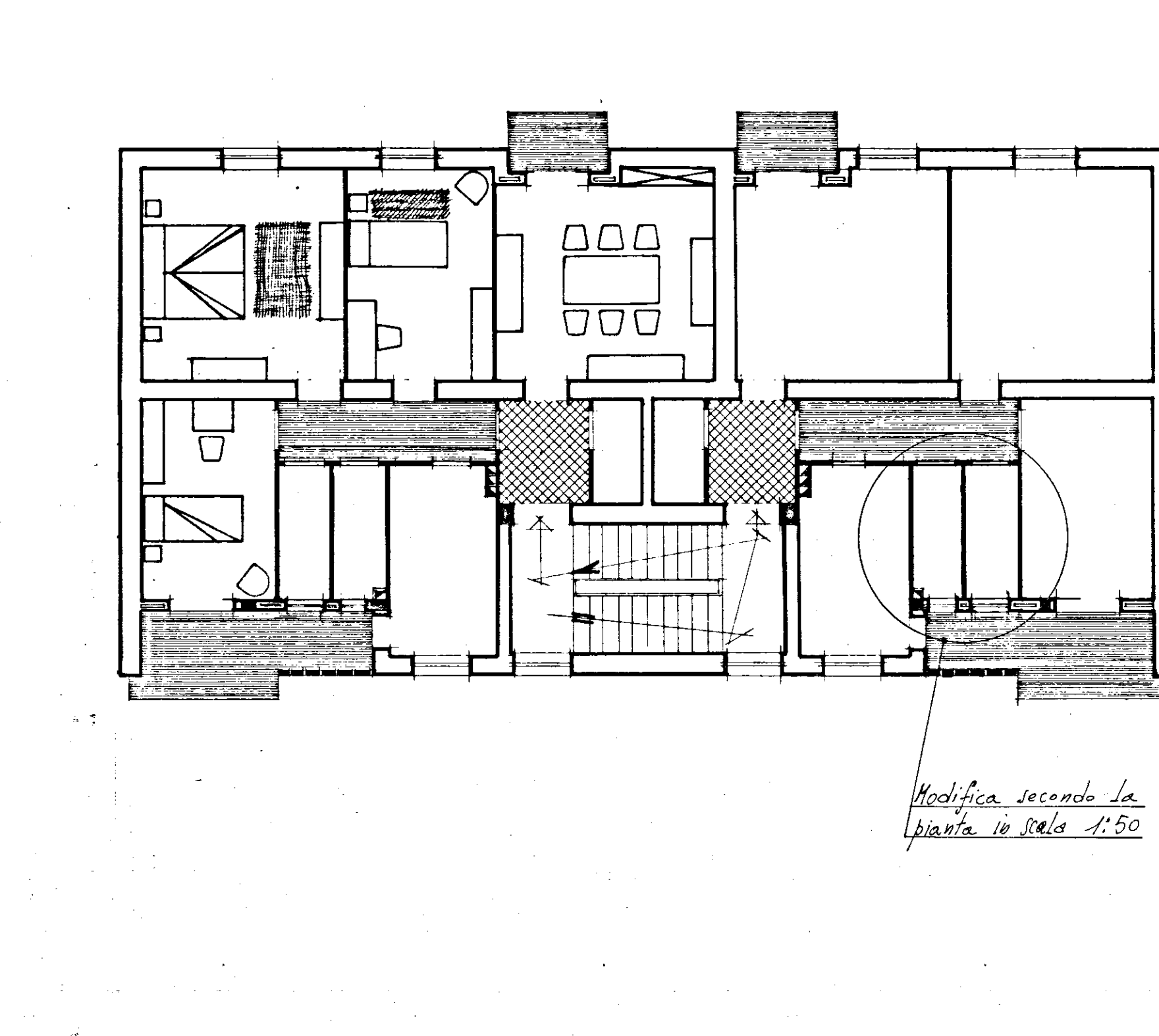
PIANO TIPO
