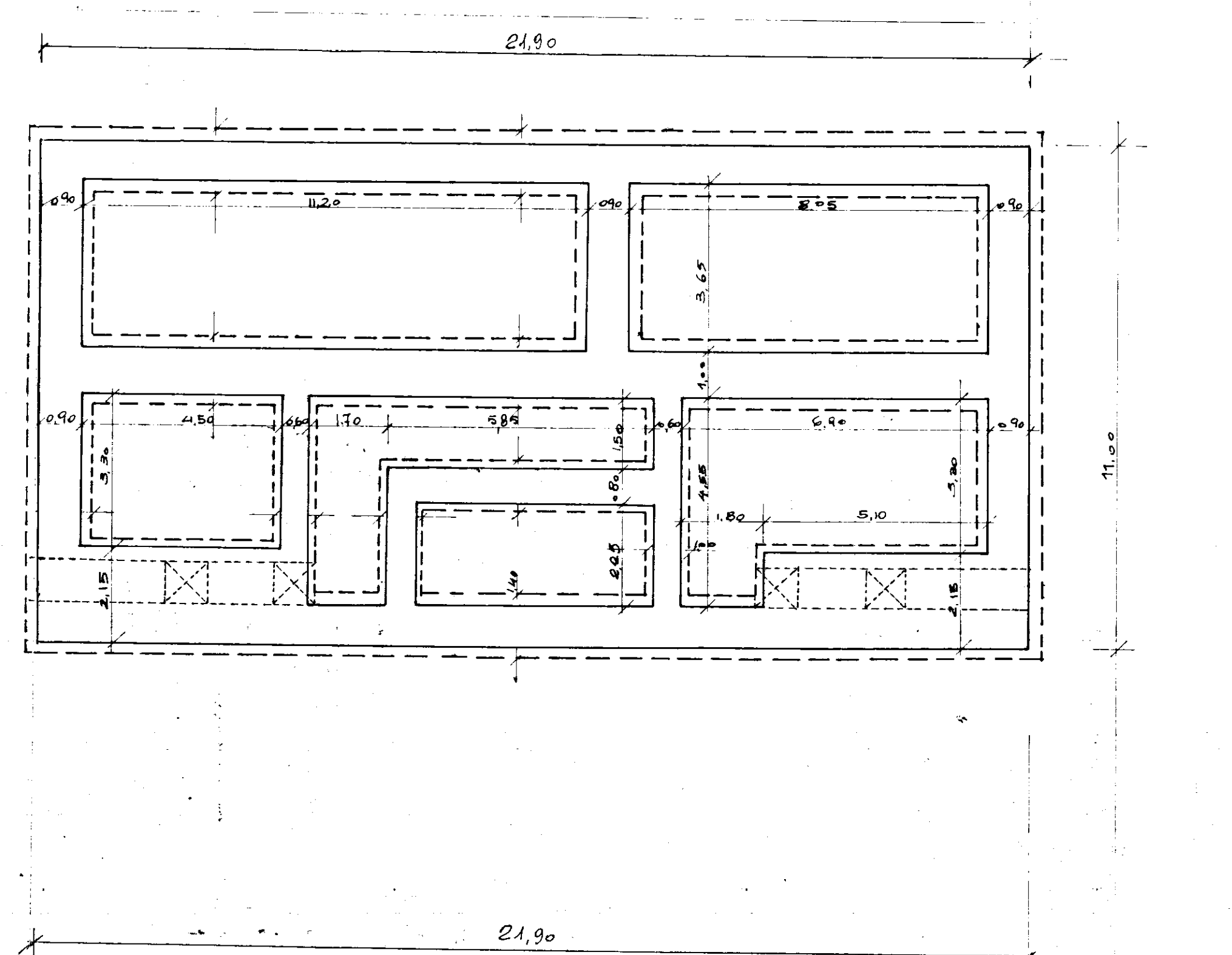
PIANTA FONDAZIONI
