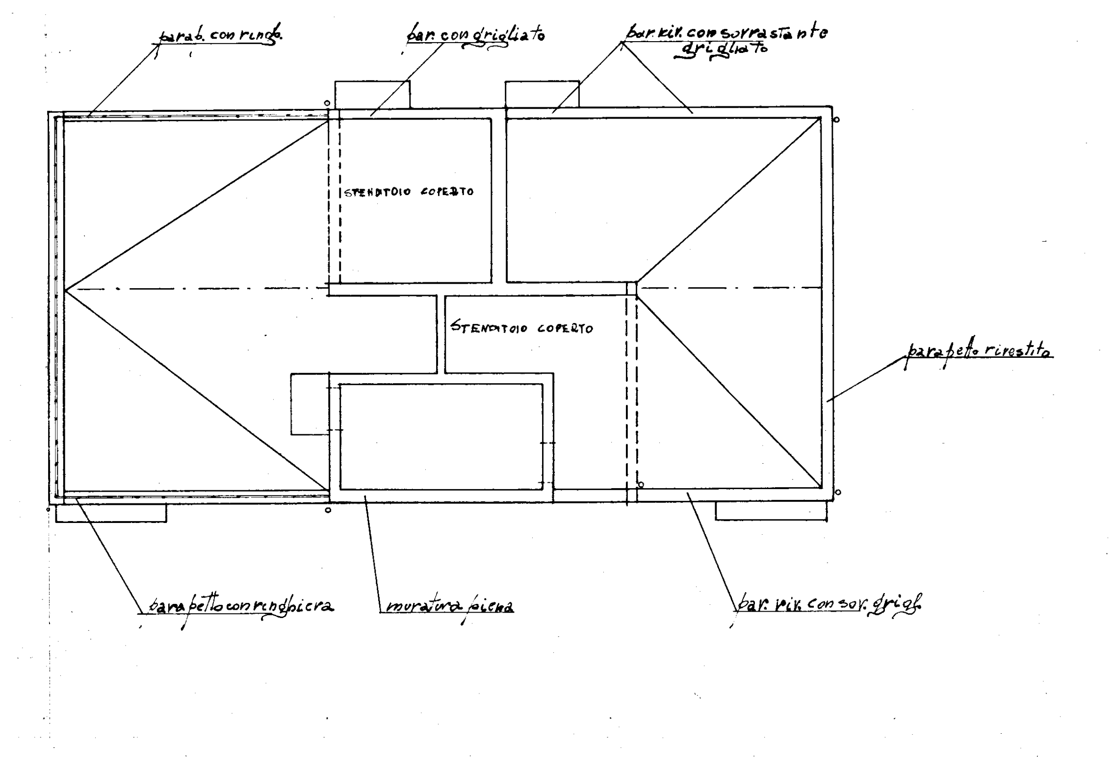
PIANTA TERRAZZA
