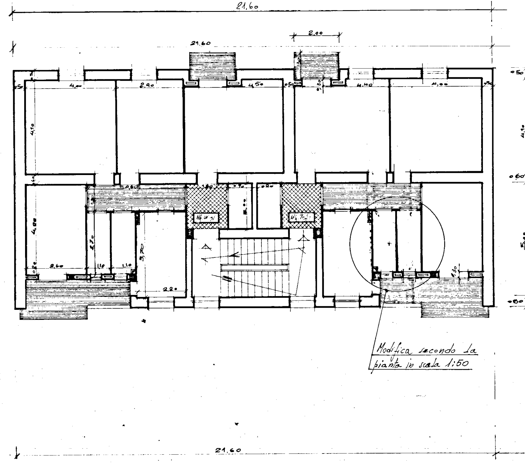
PRIMO PIANO
