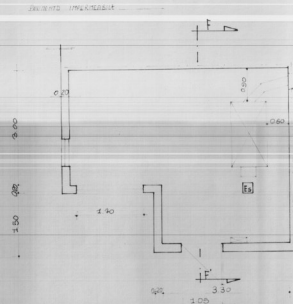
RILIEVO PIANTE CENTRALE TERMICA
