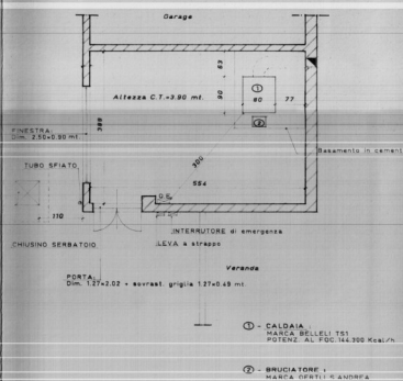
PIANTA LOCALE CENTRALE TERMICA (SCALA: 1/50)
